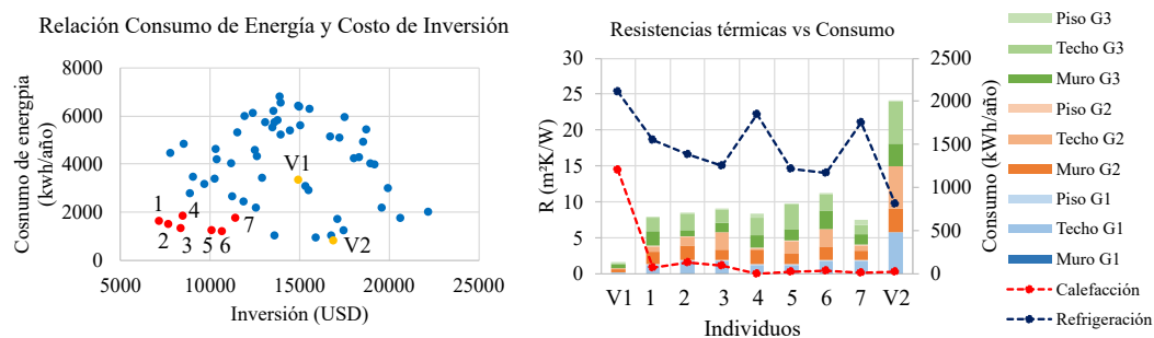
Figura 8.11: Relación entre el CI y el consumo E_{total} para Iguazu (Zona Ib)
