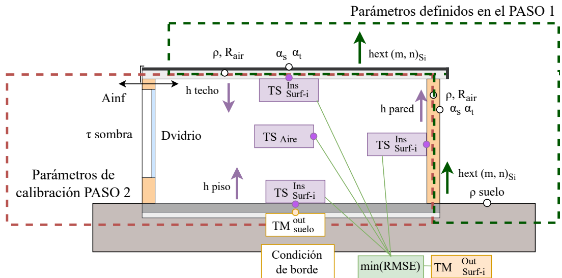
Figura 5.16: Paso 2 de la metodología escalonada propuesta: calibración del balance global.
