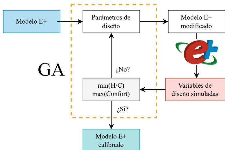
Figura 2.9: Esquema del modelo directo para el diseño óptimo de envolventes.
