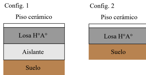
Figura 8.6: Configuraciones de aislamiento en pisos en contacto con el suelo.
