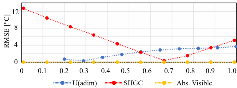
Figura 5.11: Análisis de sensibilidad del RMSE ante variaciones de U , SHGC y absorptividad visible en las superficies vidriadas.
