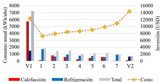
Figura 8.22: Análisis de CI y consumo E_{cal} y E_{ref} anual para Mendoza (Zona IVa)
