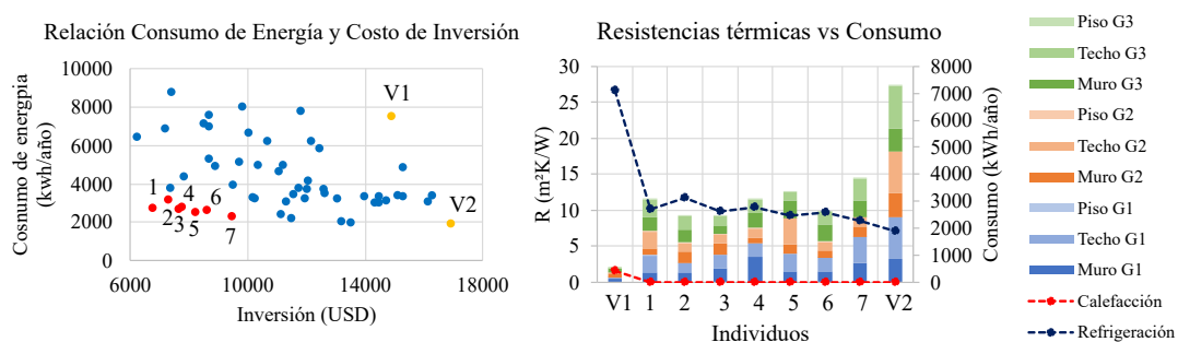
Figura 8.9: Relación entre el CI y el consumo E_{total} para Rivadavia (Zona Ia)
