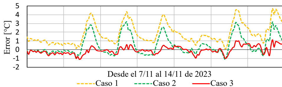
Figura 4.9: errores de Temperatura de Techo Interior para los tres casos evaluados en el Edificio MEVIR.
