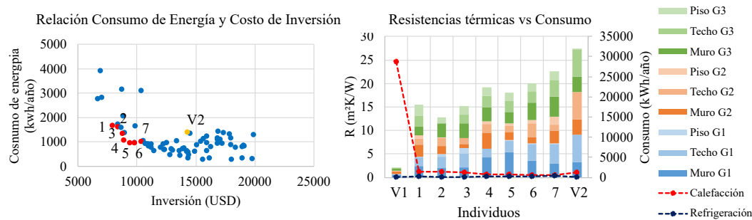
Figura 8.27: Relación entre el CI y el consumo E_{total} para San Carlos de Bariloche (Zona VI)
