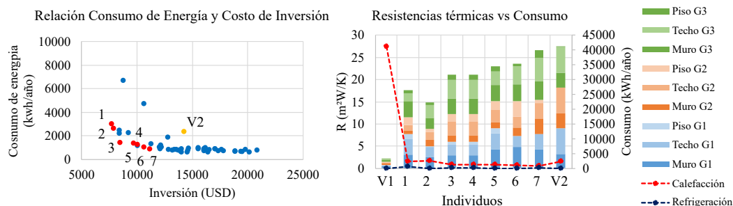
Figura 8.29: Relación entre el CI y el consumo E_{total} para Ushuaia (Zona VI)
