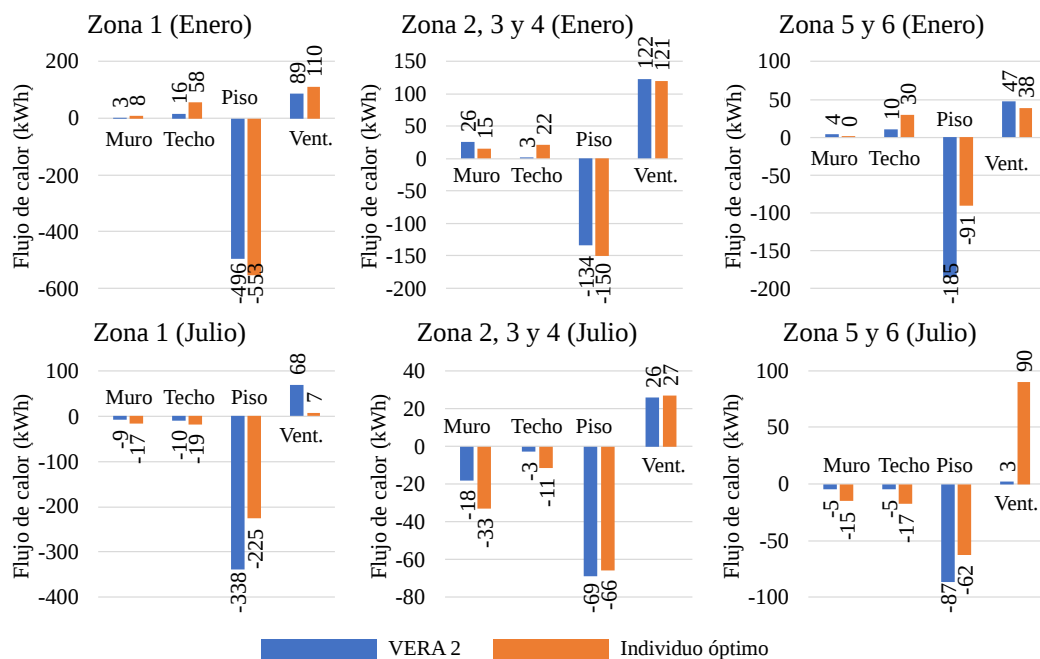
Figura 8.32: Balance térmico en Enero y Julio para Iguazú (Zona Ib)
