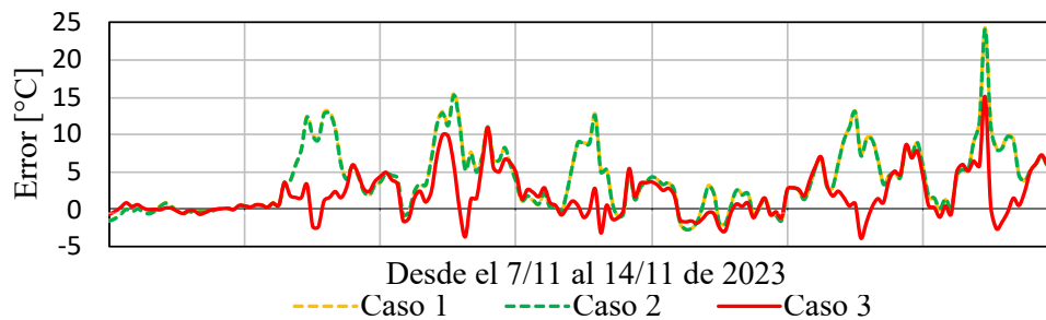
Figura 4.10: errores de Temperatura de Techo Exterior para los tres casos evaluados en el Edificio MEVIR.
