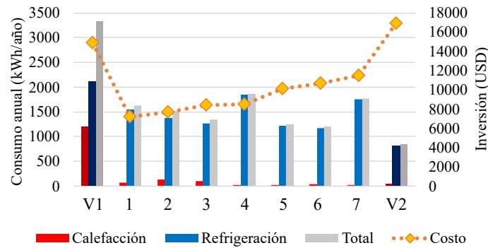
Figura 8.12: Análisis de CI y consumo E_{cal} y E_{ref} anual para Iguazú (Zona Ib)
