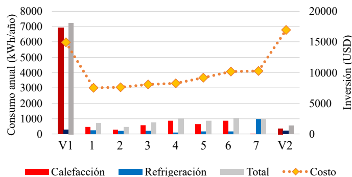
Figura 8.14: Análisis de CI y consumo E_{cal} y E_{ref} anual para Chilecito (Zona IIa)
