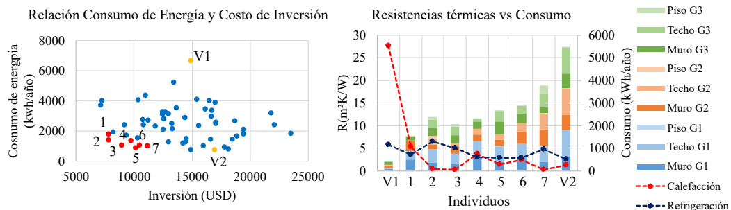
Figura 8.19: Relación entre el CI y el consumo E_{total} para Ezeiza (Zona IIIb)
