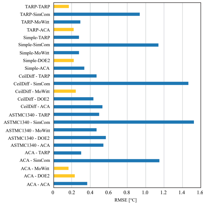
Figura 5.10: Análisis de sensibilidad del RMSE ante la variación de los modelos de coeficientes h_{int} y h_{ext} en el Edificio SOFIA.
