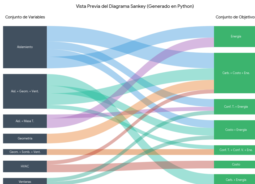
Figura 7.4: Diagrama de flujo que relaciona los conjuntos de variables de entrada con los objetivos de optimización multiobjetivo identificados.
