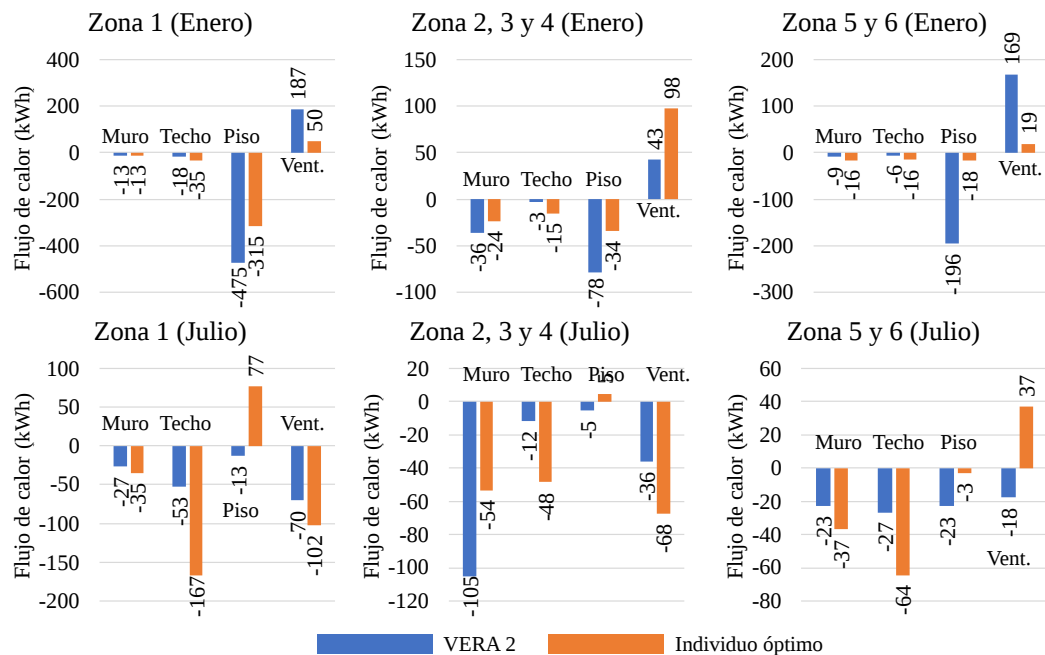
Figura 8.40: Balance térmico en Enero y Julio para San Carlos de Bariloche (Zona VI)
