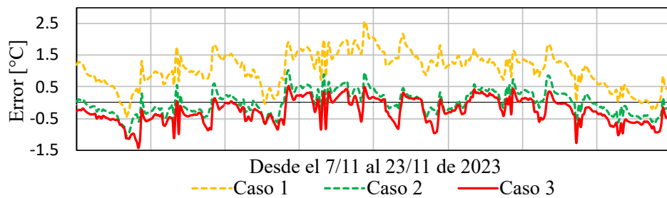
Figura 4.8: errores de Temperatura de Aire para los tres casos evaluados en el Edificio MEVIR.
