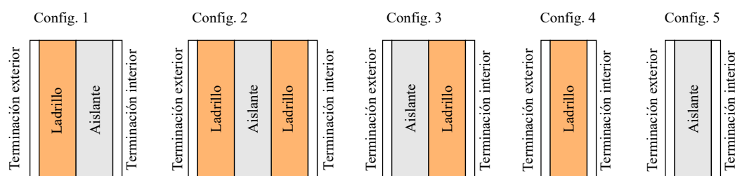
Figura 8.4: Configuraciones de capas y posición del aislante en muros del prototipo VERA.
