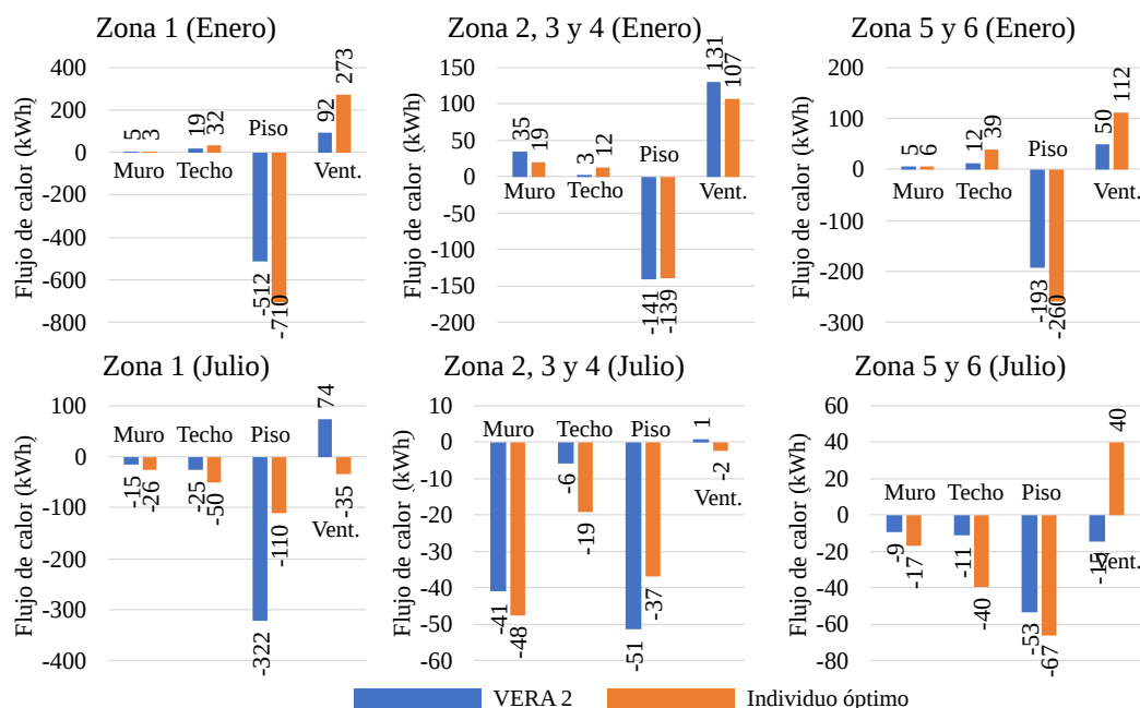
Figura 8.34: Balance térmico en Enero y Julio para Sauce Viejo (Zona IIB)
