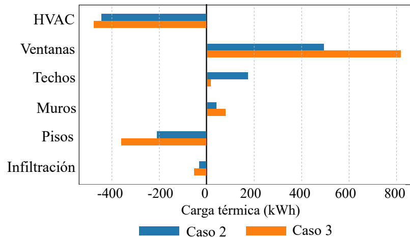
Figura 4.16: Cargas térmicas durante el periodo estival en el Edificio MEVIR.
