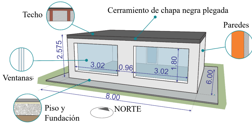
Figura 5.2: Geometría y materiales del Edificio SOFIA.
