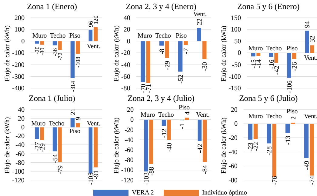
Figura 8.41: Balance térmico en Enero y Julio para Ushuaia (Zona VI)
