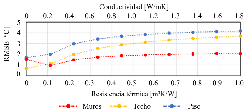
Figura 5.4: Análisis de sensibilidad del RMSE ante variaciones de la R_{aire} en las superficies opacas del Edificio SOFIA.
