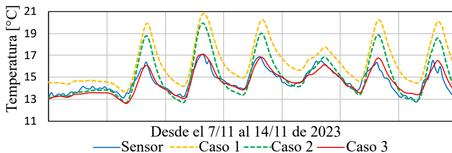
Figura 4.14: Comparativa de Temperatura de Techo Interior medida y simulada para los tres casos evaluados en el Edificio MEVIR.
