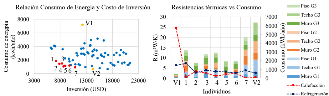
Figura 8.21: Relación entre el CI y el consumo E_{total} para Mendoza (Zona IVa)
