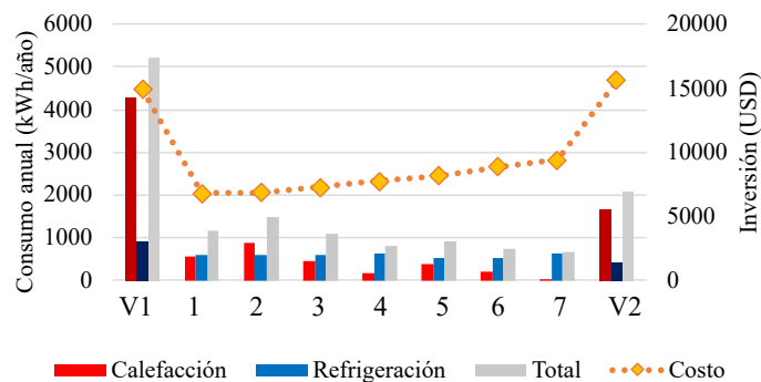
Figura 8.18: Análisis de CI y consumo E_{cal} y E_{ref} anual para Córdoba (Zona IIIa)
