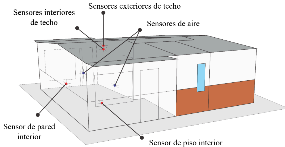
Figura 4.4: Sistema de monitoreo del Edificio MEVIR.
