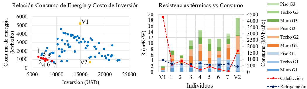
Figura 8.17: Relación entre el CI y el consumo E_{total} para Córdoba (Zona IIIa)
