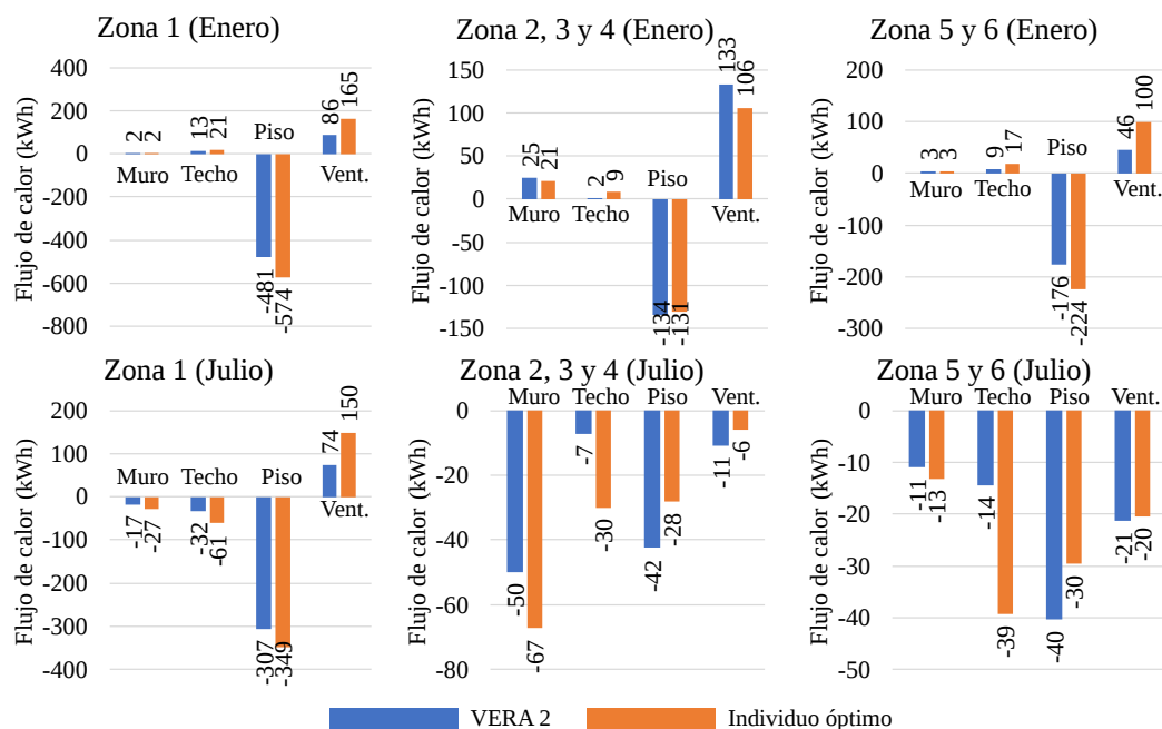
Figura 8.36: Balance térmico en Enero y Julio para Ezeiza (Zona IIIb)
