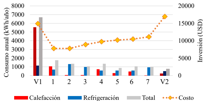
Figura 8.20: Análisis de CI y consumo E_{cal} y E_{ref} anual para Ezeiza (Zona IIIb)
