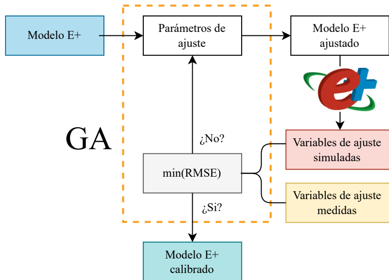
Figura 2.8: Esquema del modelo inverso aplicado a la calibración de modelos BES .
