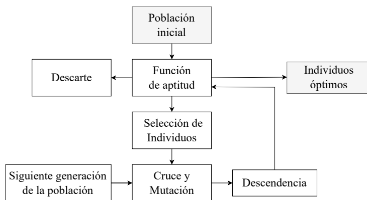
Figura 2.7: Diagrama de flujo del algoritmo GA .
