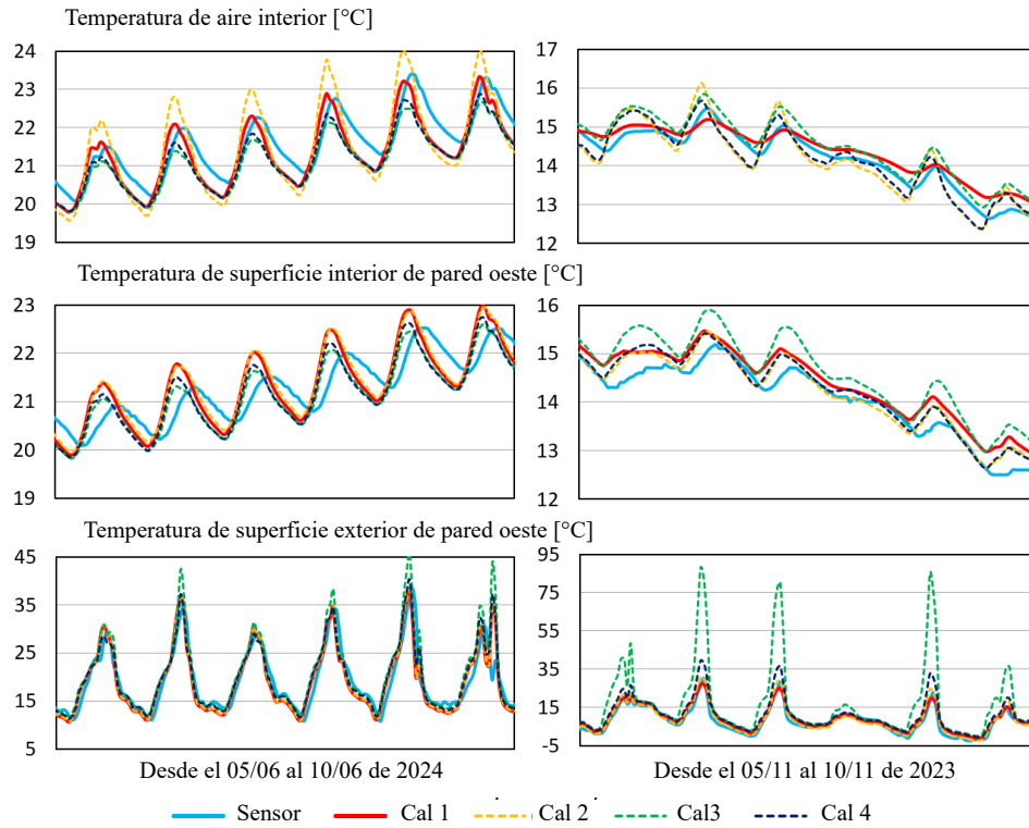
Figura 5.26: Resultados del cruce de parámetros estacional (Verano vs. Invierno).
