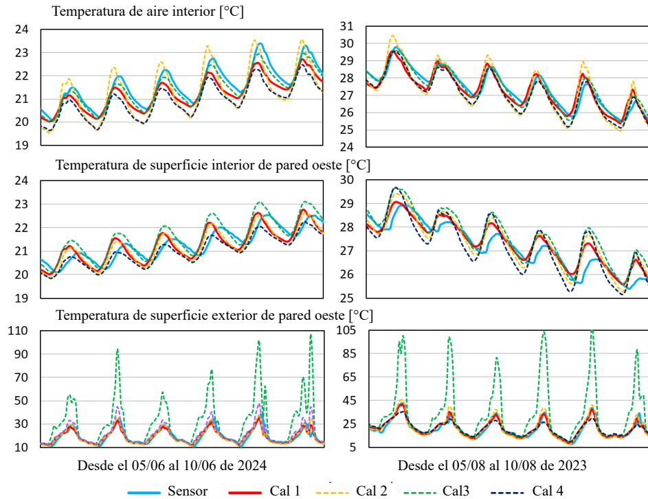
Figura 5.25: Temperaturas resultantes del cruce de parámetros entre Junio y Agosto.
