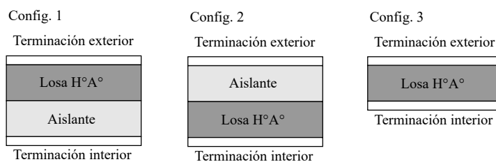
Figura 8.5: Configuraciones de montaje y posición del aislante en cubiertas.
