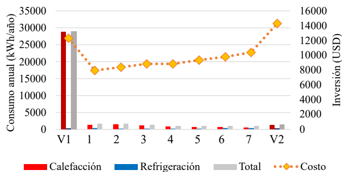
Figura 8.28: Análisis de CI y consumo E_{cal} y E_{ref} anual para San Carlos de Bariloche (Zona VI)
