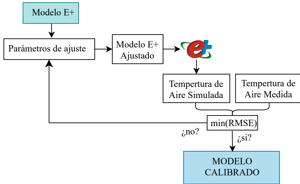
Figura 5.18: Metodología de calibración Mono-Objetivo.
