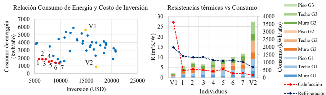
Figura 8.15: Relación entre el CI y el consumo E_{total} para Sauce Viejo (Zona IIb)
