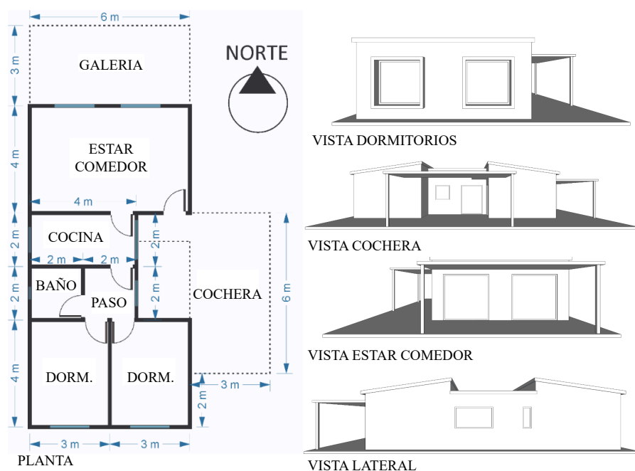
Figura 8.1: Zonificación funcional y esquema arquitectónico del prototipo VERA.
