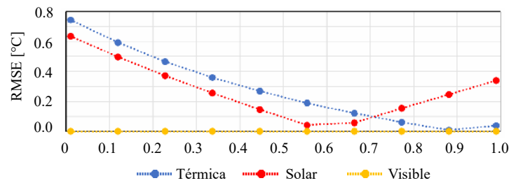
Figura 5.5: Análisis de sensibilidad del RMSE ante variaciones de \alpha_S y \alpha_T en el techo del Edificio SOFIA.
