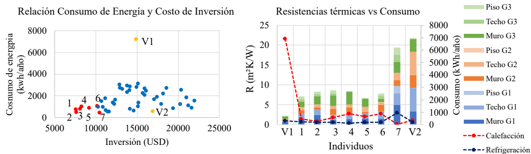
Figura 8.13: Relación entre el CI y el consumo E_{total} para Chilecito (Zona IIa)
