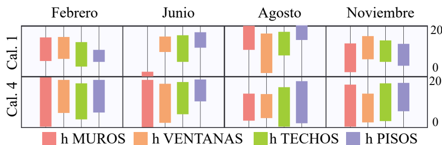
Figura 5.29: Dispersión del coeficiente convectivo interior (Rango: 0.00–20.00 W/m^2 K ).
