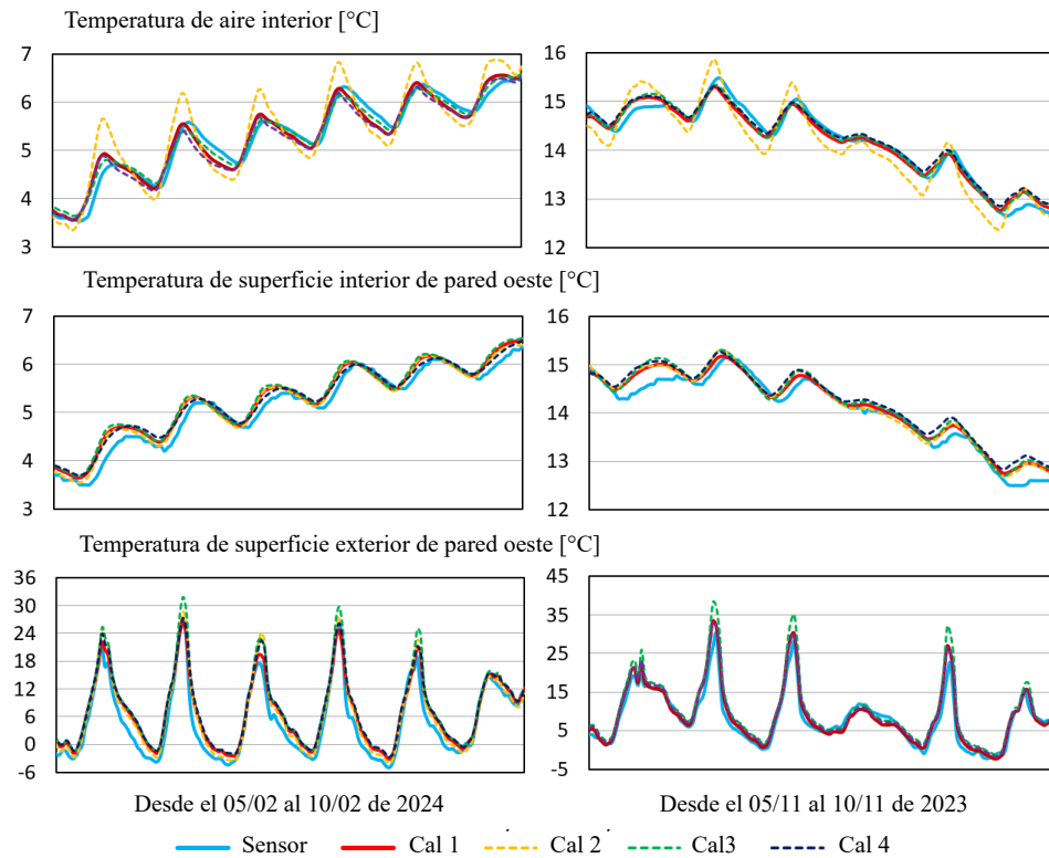
Figura 5.24: Temperaturas resultantes del cruce de parámetros entre Febrero y Noviembre.
