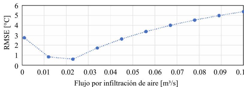
Figura 5.12: Análisis de sensibilidad del RMSE ante variaciones del Q_{inf} en el Edificio SOFIA.
