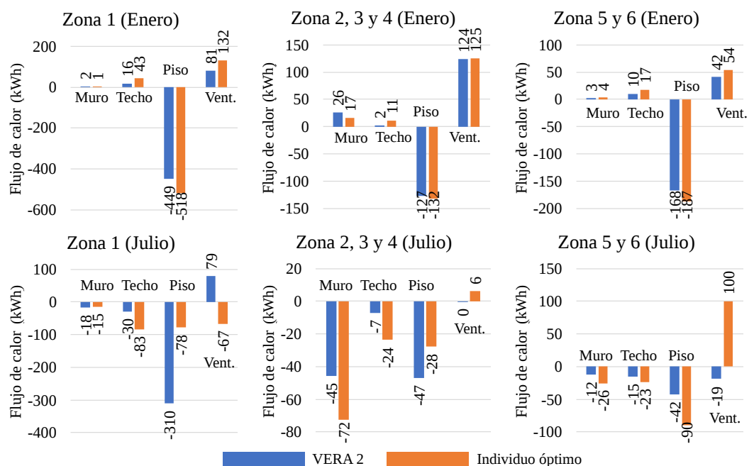
Figura 8.35: Balance térmico en Enero y Julio para Córdoba (Zona IIIa)
