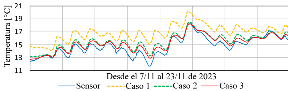
Figura 4.12: Comparativa de Temperatura de Muro Interior medida y simulada para los tres casos evaluados en el Edificio MEVIR.
