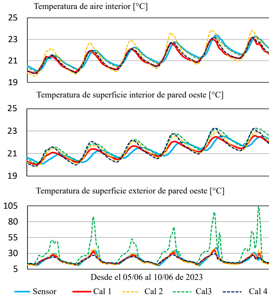
Figura 5.21: Temperaturas resultantes de las distintas calibraciones en el mes de junio.
