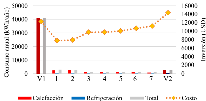
Figura 8.30: Análisis de CI y consumo E_{cal} y E_{ref} anual para Ushuaia (Zona VI)
