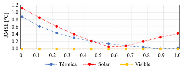
Figura 5.7: Análisis de sensibilidad del RMSE ante variaciones de \alpha_S y \alpha_T en el piso del Edificio SOFIA.
