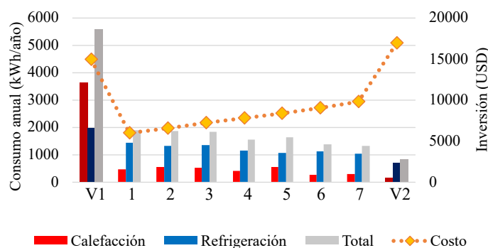
Figura 8.16: Análisis de CI y consumo E_{cal} y E_{ref} anual para Sauce Viejo (Zona IIb)
