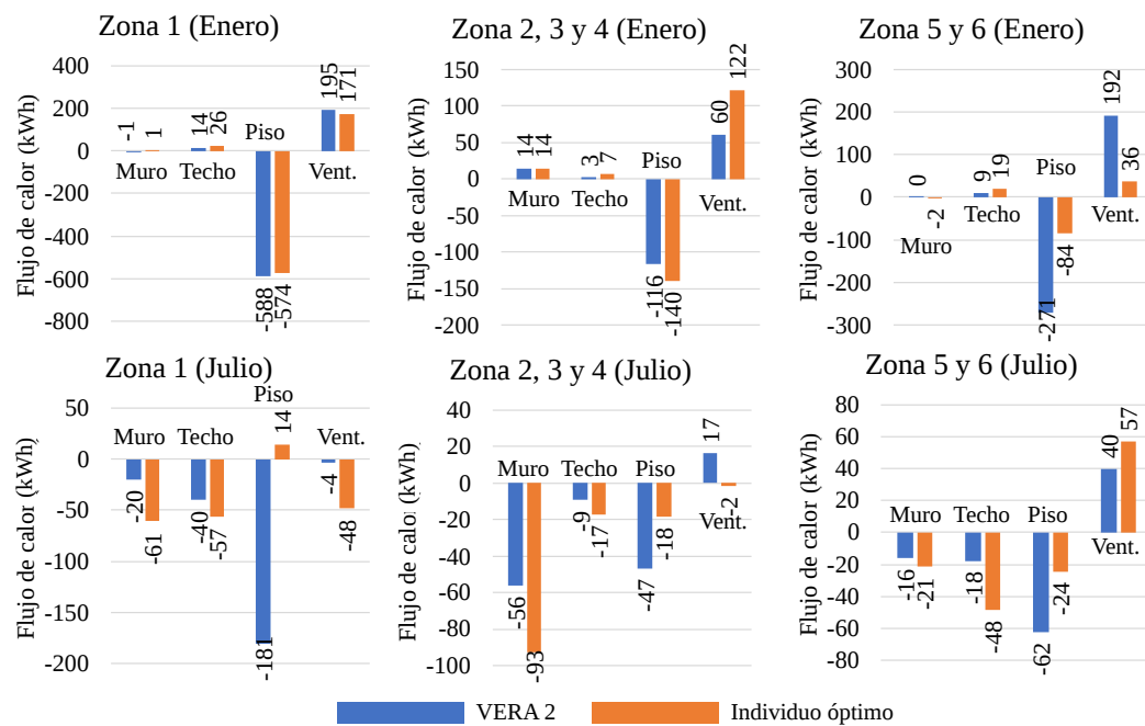
Figura 8.37: Balance térmico en Enero y Julio para Mendoza (Zona IVa)
