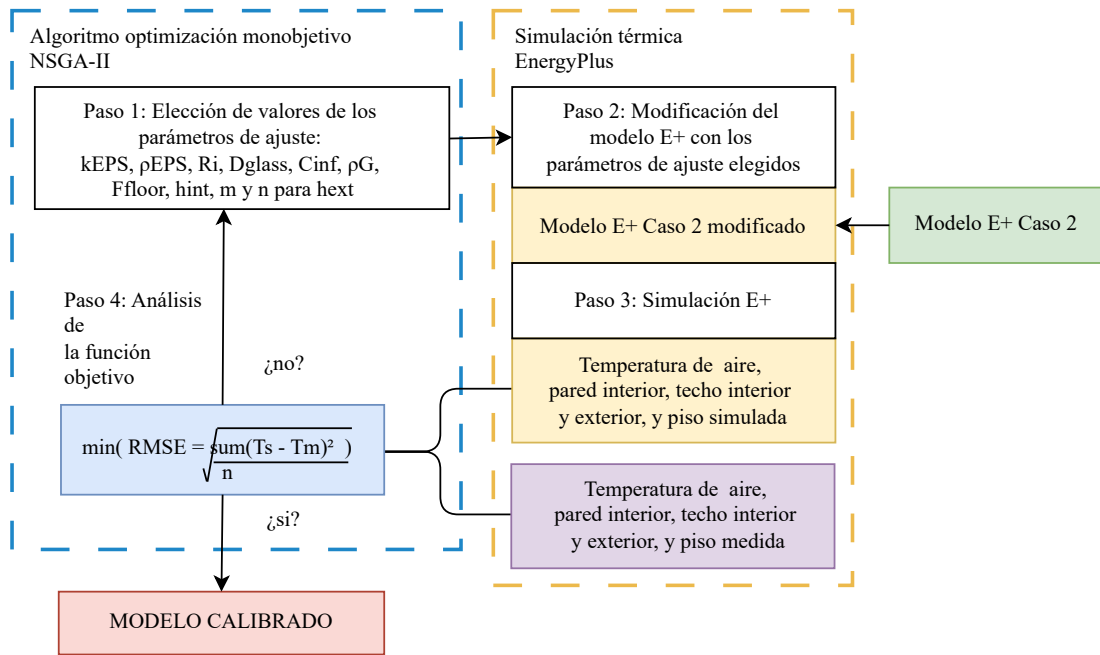
Figura 4.7: Caso 3: Pseudocódigo de Calibración Multi-objetivo Edificio MEVIR.
