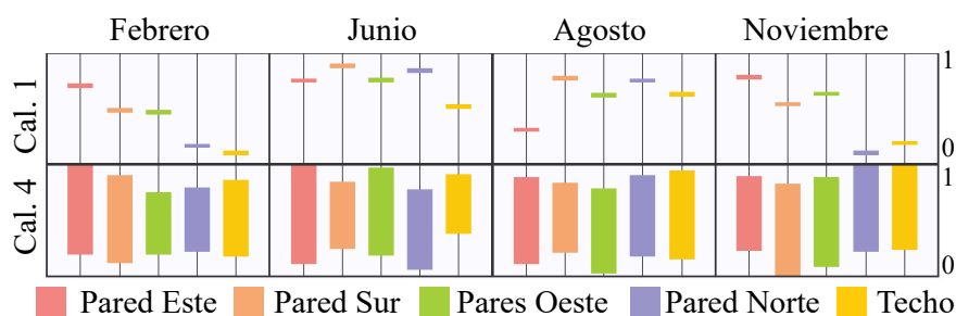
Figura 5.28: Dispersión de la resistencia térmica del aire R_{aire} (Rango: 0.00–1.00 m^2 K/W ).
