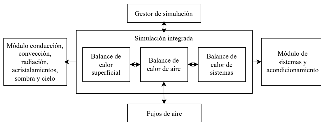
Figura 2.2: Arquitectura de simulación integrada de E+ : interacción entre los balances de calor de superficie, aire y sistemas.
