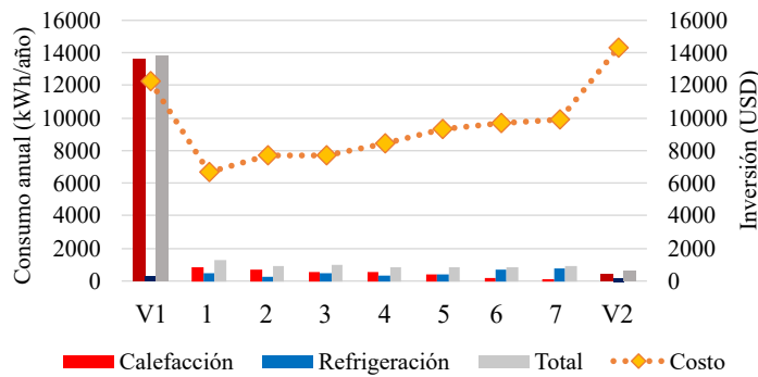
Figura 8.26: Análisis de CI y consumo E_{cal} y E_{ref} anual para Comodoro Rivadavia (Zona V)
