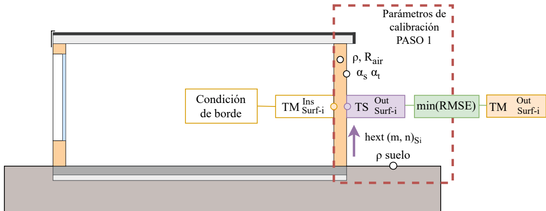
Figura 5.15: Paso 1 de la metodología escalonada propuesta: aislamiento de componentes opacos.
