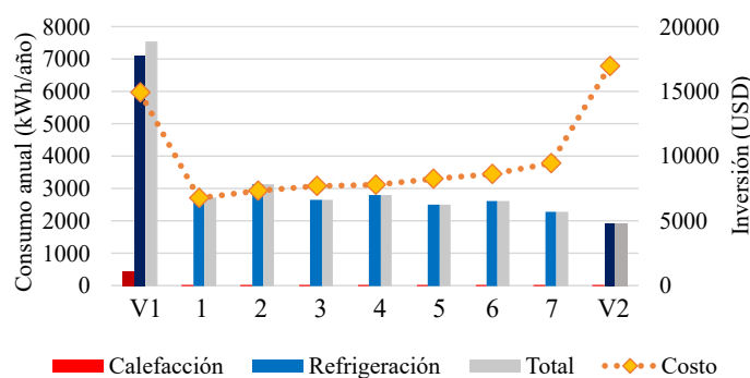
Figura 8.10: Análisis de CI y consumo E_{cal} y E_{ref} anual para Rivadavia (Zona Ia)
