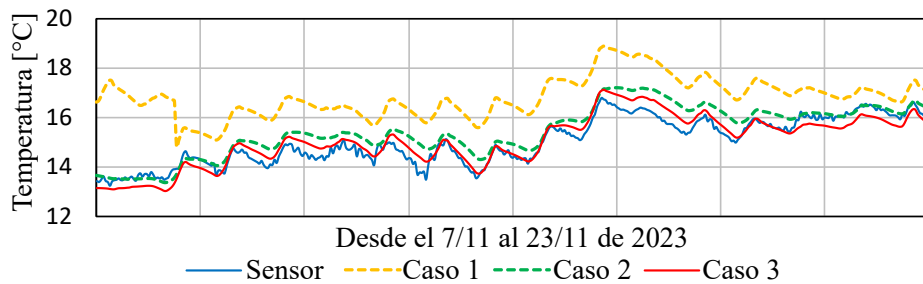
Figura 4.13: Comparativa de Temperatura de Piso Interior medida y simulada para los tres casos evaluados en el Edificio MEVIR.
