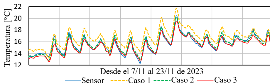
Figura 4.11: Comparativa de Temperatura de Aire medida y simulada para los tres casos evaluados en el Edificio MEVIR.
