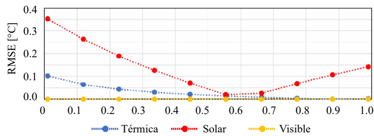
Figura 5.9: Análisis de sensibilidad del RMSE ante variaciones de \alpha_S y \alpha_T en la superficie exterior de muros del Edificio SOFIA.
