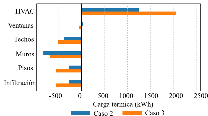
Figura 4.17: Cargas térmicas durante el periodo invernal en el Edificio MEVIR.
