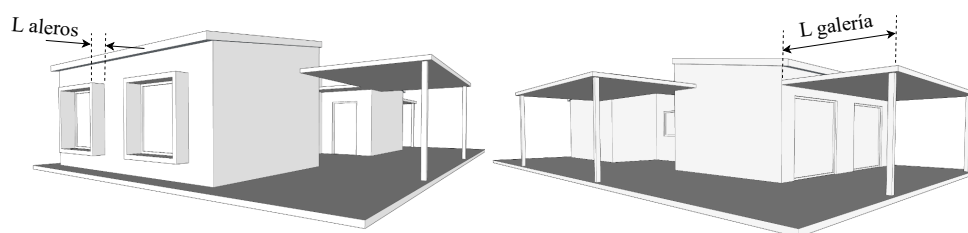
Figura 8.7: Dimensiones de aleros y galerías.
