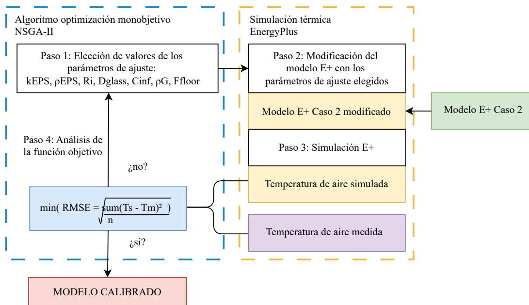
Figura 4.6: Caso 2 : Pseudocódigo de Calibración Mono-Objetivo Edificio MEVIR.
