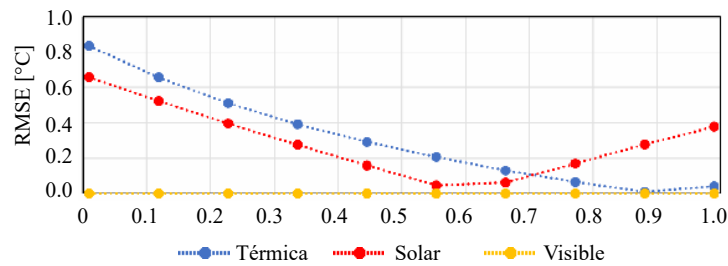
Figura 5.8: Análisis de sensibilidad del RMSE ante variaciones de \alpha_S y \alpha_T en la superficie interior de muros del Edificio SOFIA.
