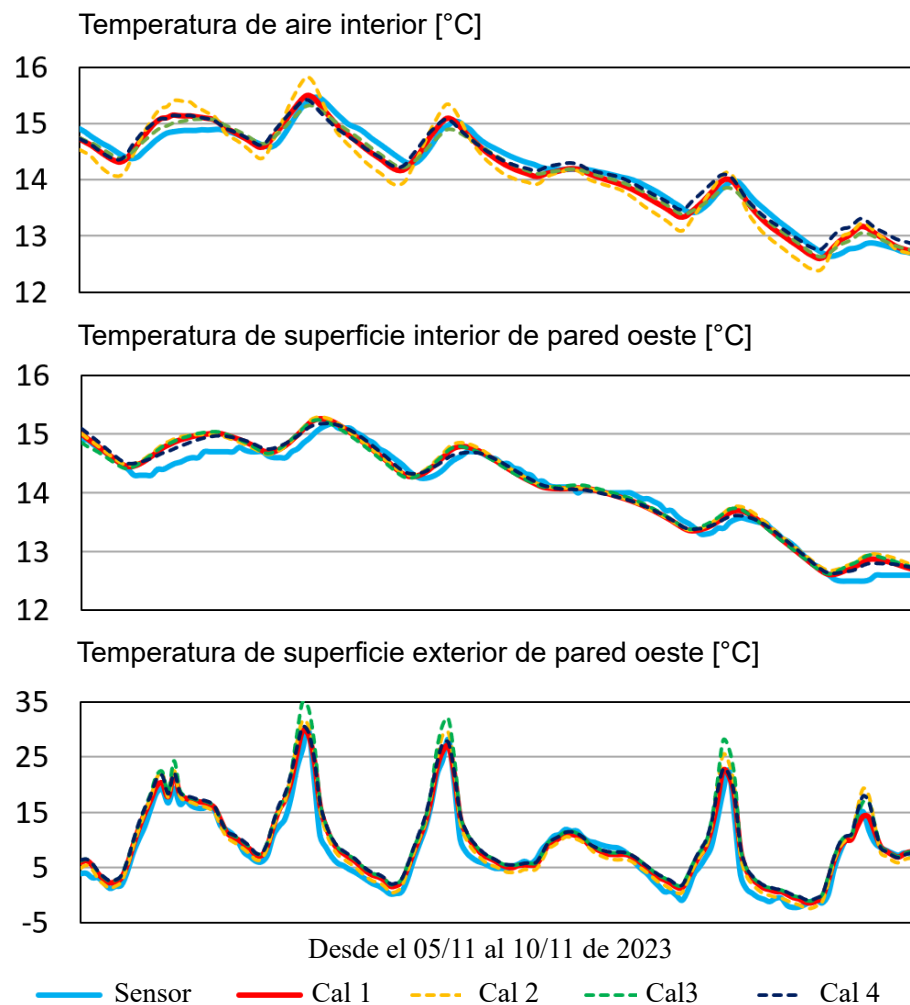
Figura 5.23: Evolución de temperaturas en el mes de noviembre.
