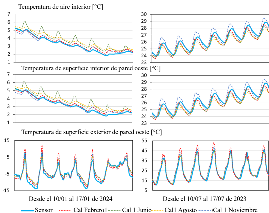
Figura 5.27: Temperaturas resultantes de la validación en los meses de Enero y Julio.
