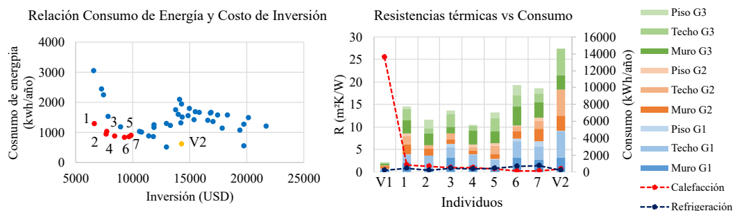
Figura 8.25: Relación entre el CI y el consumo E_{total} para Comodoro Rivadavia (Zona V)
