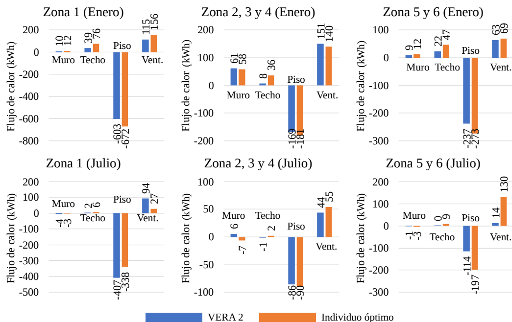
Figura 8.31: Balance térmico en Enero y Julio para Rivadavia (Zona Ia)
