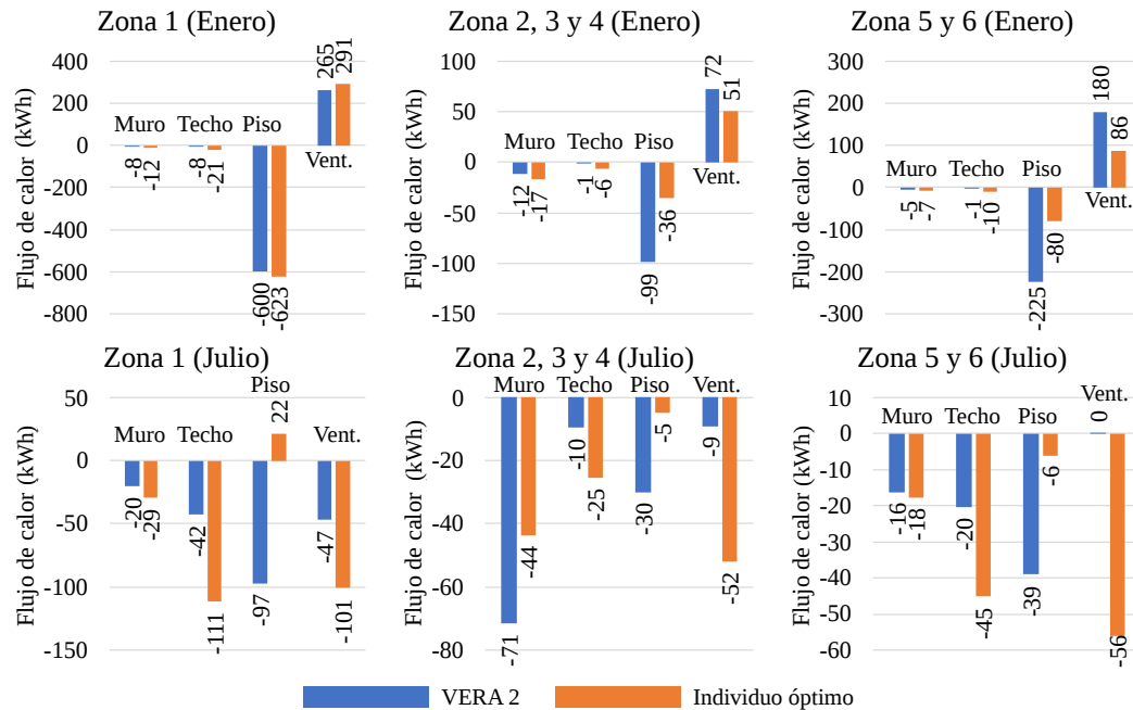
Figura 8.39: Balance térmico en Enero y Julio para Comodoro Rivadavia (Zona V)
