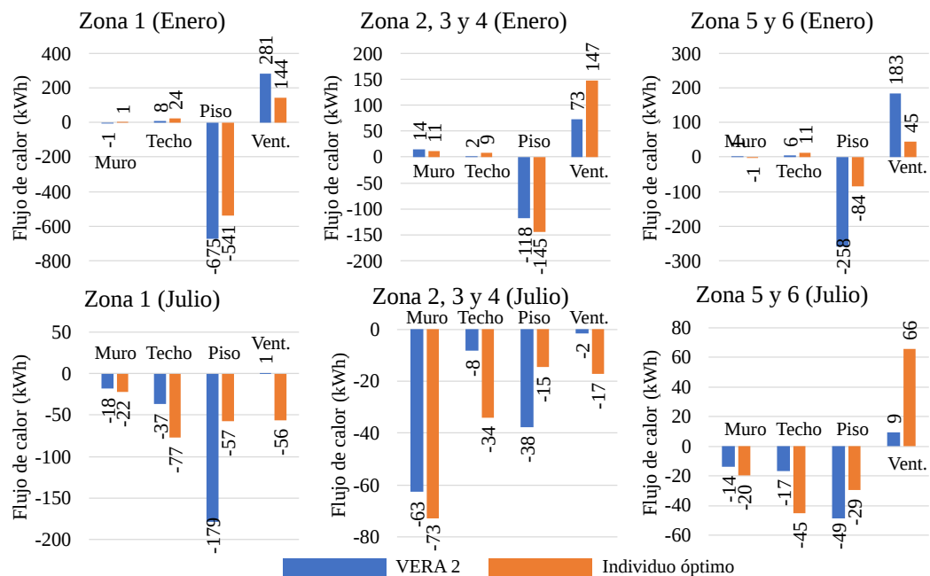
Figura 8.38: Balance térmico en Enero y Julio para Bahía Blanca (Zona IVb)
