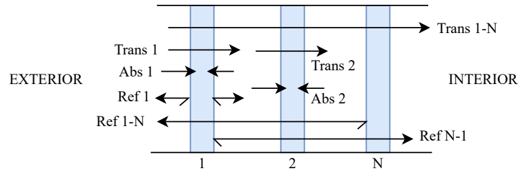
Figura 2.6: Esquema del balance de calor en elementos transparentes mediante el enfoque de nodos múltiples.
