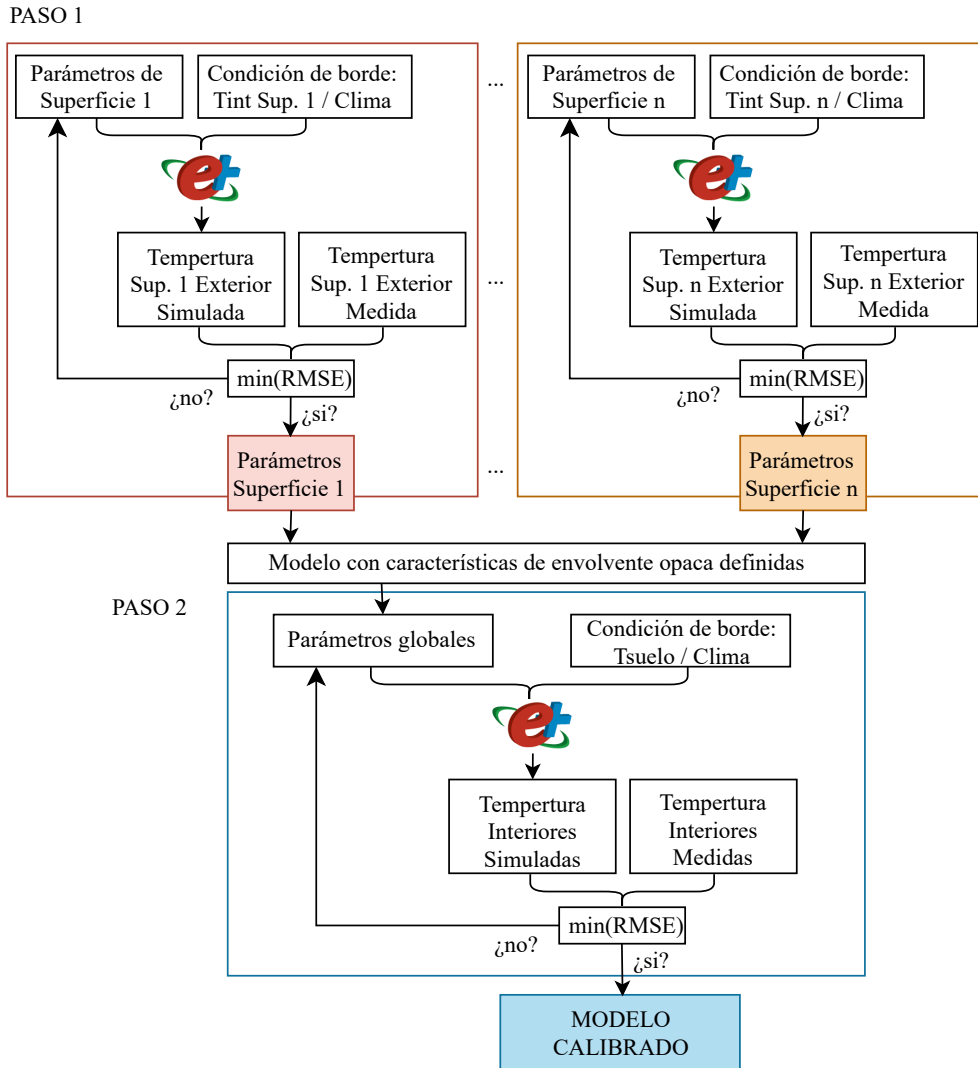
Figura 5.17: Metodología de calibración en dos pasos ( Step-wise ) para el Edificio SOFIA.
