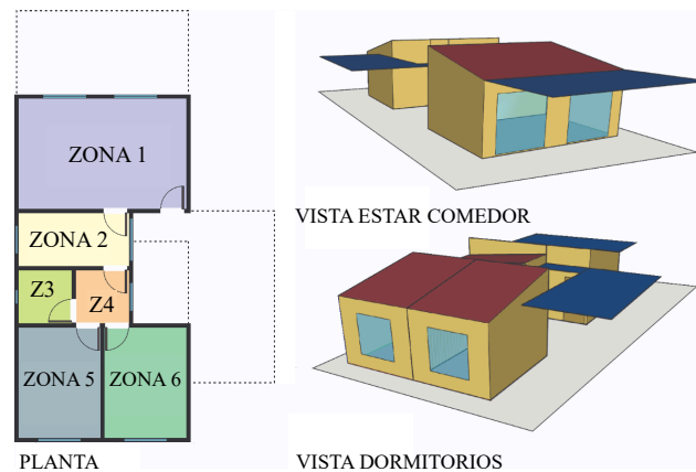
Figura 8.2: Zonificación térmica y modelo computacional del prototipo VERA en E+ .
