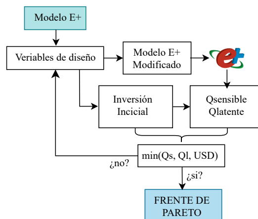
Figura 8.3: Acople entre E+ y NSGA-II para el diseño óptimo de envolvente del prototipo VERA.
