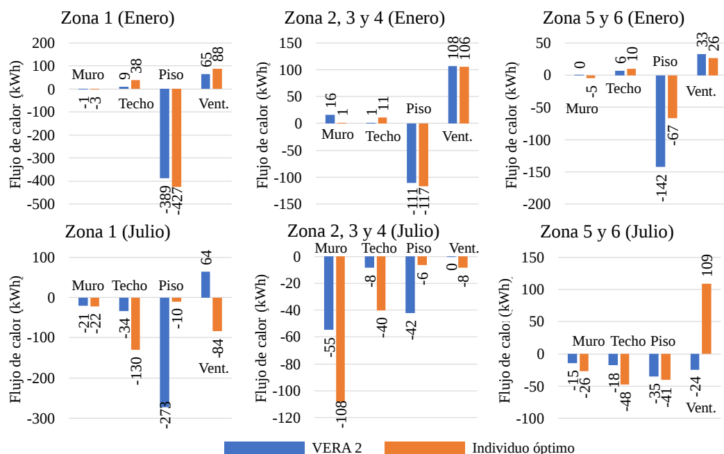
Figura 8.33: Balance térmico en Enero y Julio para Chilecito (Zona IIa)
