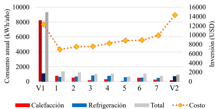
Figura 8.24: Análisis de CI y consumo E_{cal} y E_{ref} anual para Bahía Blanca (Zona IVb)
