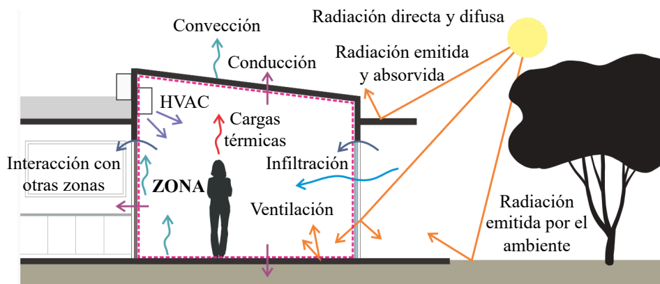
Figura 2.1: Esquema de los mecanismos de transferencia de calor y masa que intervienen en el balance energético de una zona térmica.
