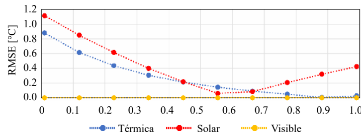
Figura 5.6: Análisis de sensibilidad del RMSE ante variaciones de \alpha_S y \alpha_T en el cielorraso del Edificio SOFIA.
