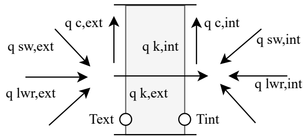
Figura 2.5: Esquema de los componentes del balance de calor superficial en un elemento opaco de la envolvente.
