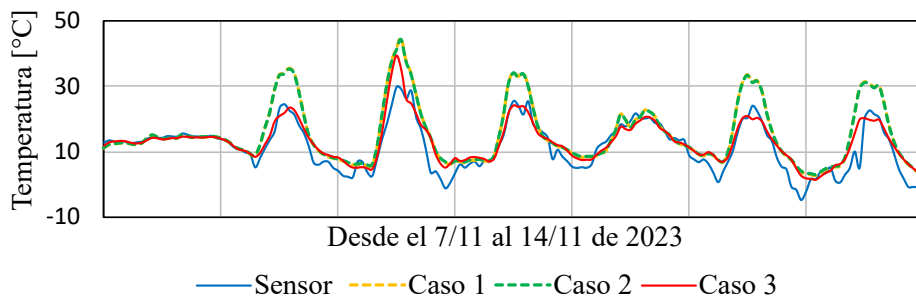
Figura 4.15: Comparativa de Temperatura de Techo Exterior medida y simulada para los tres casos evaluados en el Edificio MEVIR.
