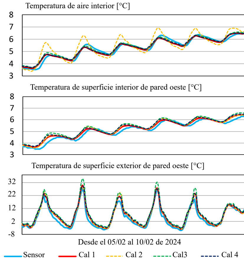
Figura 5.20: Temperaturas resultantes de las distintas calibraciones en el mes de febrero.
