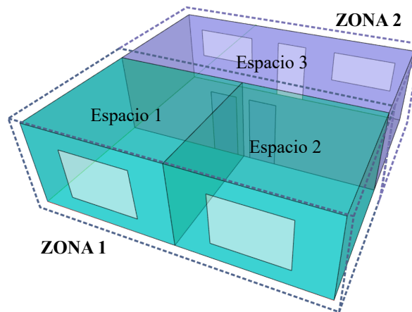
Figura 2.4: Estrategia de zonificación térmica: agrupación de múltiples espacios físicos en volúmenes de control homogéneos para la simulación energética.
