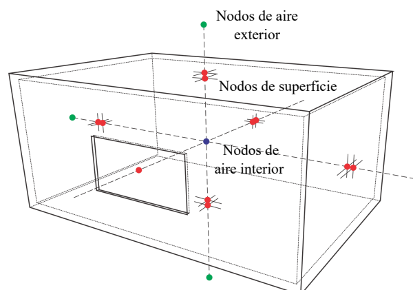
Figura 2.3: Representación esquemática de la red nodal de una zona térmica para la aplicación del método de balance de calor.
