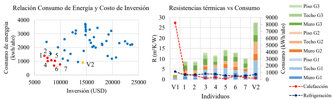
Figura 8.23: Relación entre el CI y el consumo E_{total} para Bahía Blanca (Zona IVb)
