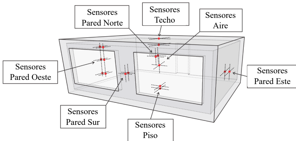
Figura 5.3: Sistema de monitoreo del Edificio SOFIA.
