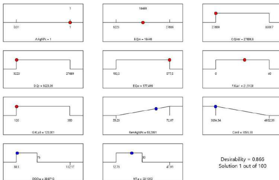
Figura A.14 - Optimización numérica de la función de deseabilidad utilizando RSM para el Escenario 4-B, BSM1 modificado. AgNPS: 1 mgAg/L, Qin: 18446 m 3 /d.
