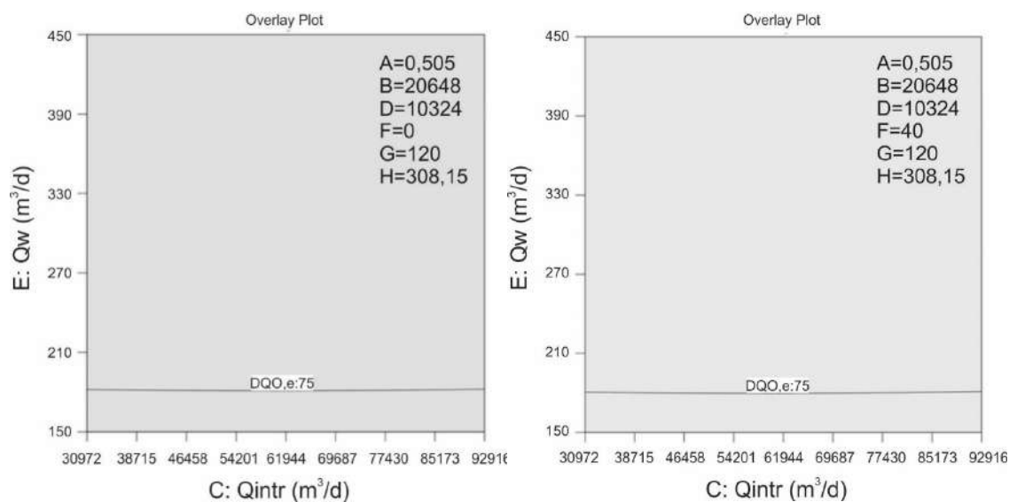
Figura A.29 - Zona óptima de las respuestas analizadas para el modelo BSM2 modificado. Escenario 3. Remoción de AgNPs 60%. Factores C: Qintr y E: Qw. A: 0,505mgAg/L, B: 20648 m³/d, D: 10324 m³/d, G: 120 l/d, H: 308,15 K. En a) F: 0 l/d, b) F: 40 l/d.
