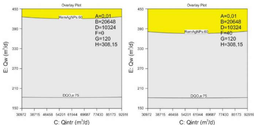
Figura A.23 - Zona óptima de las respuestas analizadas para el modelo BSM2 modificado. Escenario 1. Remoción de AgNPs 60%. Factores C: Qintr y E: Qw. A: 0,01 mgAg/L, B: 20648 m³/d, D: 10324 m³/d, G: 120 1/d, H: 308,15 K. En a) F: 0 1/d, b) F: 40 1/d.
