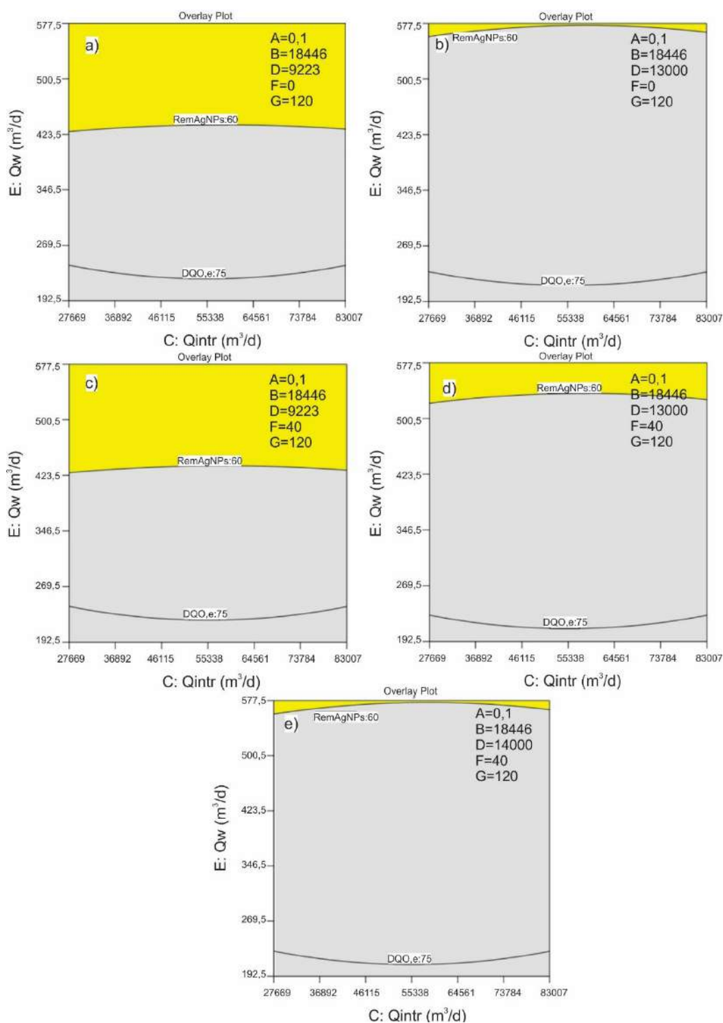
Figura 6.13 - Zona óptima de las respuestas analizadas para modelo BSM1 modificado. Remoción de AgNPs 60%. Factores C: caudal de reciclaje interno (m³/d), E: Caudal de rechazo (m³/d). A: 0,1 mgAg/L, B: 18446 m³/d, G: 120 1/d. En a) D: 9223 m³/d y F: 0 1/d, b) D: 13000 m³/d y F: 0 1/d, c) D: 9223 m³/d y F: 40 1/d, d) D: 13000 m³/d y F: 40 1/d, e) D: 14000 m³/d y F: 40 1/d.
