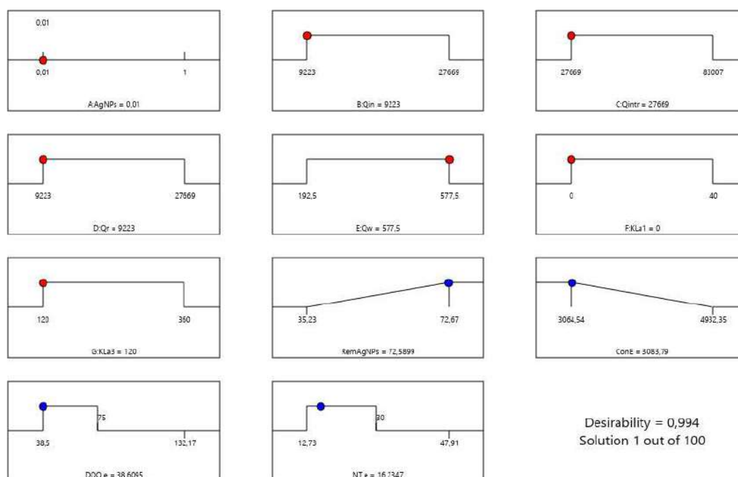
Figura A.1 - Optimización numérica para el Escenario 1-A, para el modelo BSM1 modificado. AgNPS: 0,01 mgAg/L, Qin libre. Deseabilidad: 0,994.
