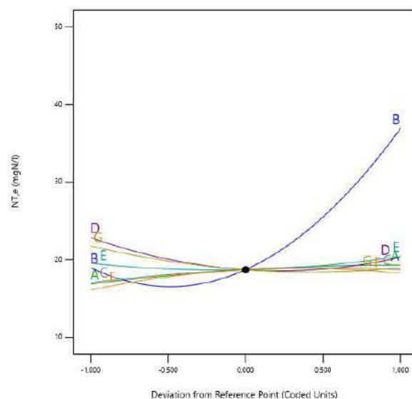
Figura 6.9- Gráfico de perturbaciones para la respuesta 'R4: NT,e' en el modelo BSM1 modificado.
