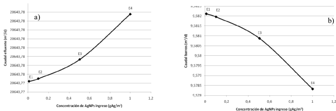
Figura 5.6 - Caudales de efluente y barros para los distintos escenarios - BSM2 modificado. a) Caudal de efluente (m³/d), b) Caudal de barros (m³/d).
