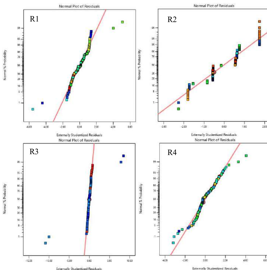
Figura 6.2 - Gráficos de residuos normales para las respuestas del modelo BSM1 modificado. R1: Remoción de AgNPs, R2: Consumo de Energía, R3: DQO efluente, R4: Nitrógeno Total efluente.
