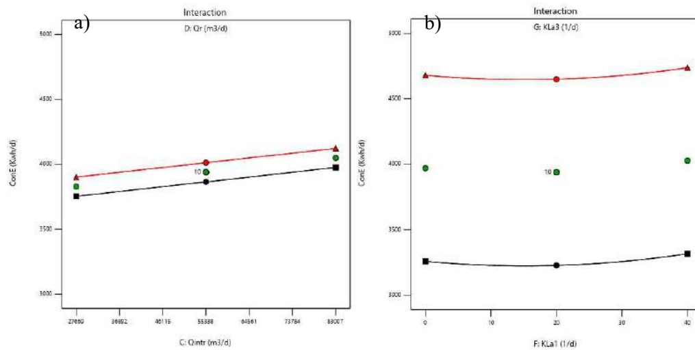
Figura 6.6 - Gráficos de las interacciones más significativas entre los factores: a) CD y b) FG, para la respuesta 'R2: ConE' en el modelo BSM1 modificado.
