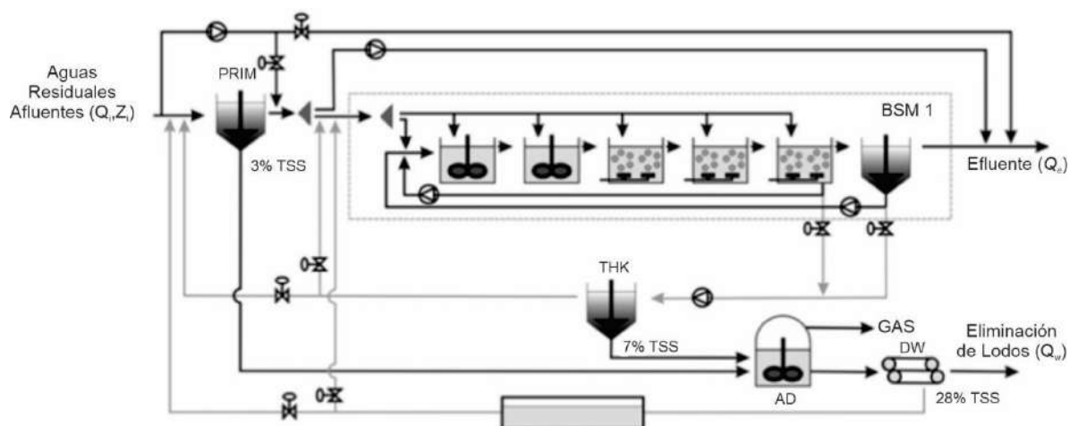
Figura 4.3 - Esquema de la planta para el modelo BSM2. Adaptado de Alex et al. (2009b).
