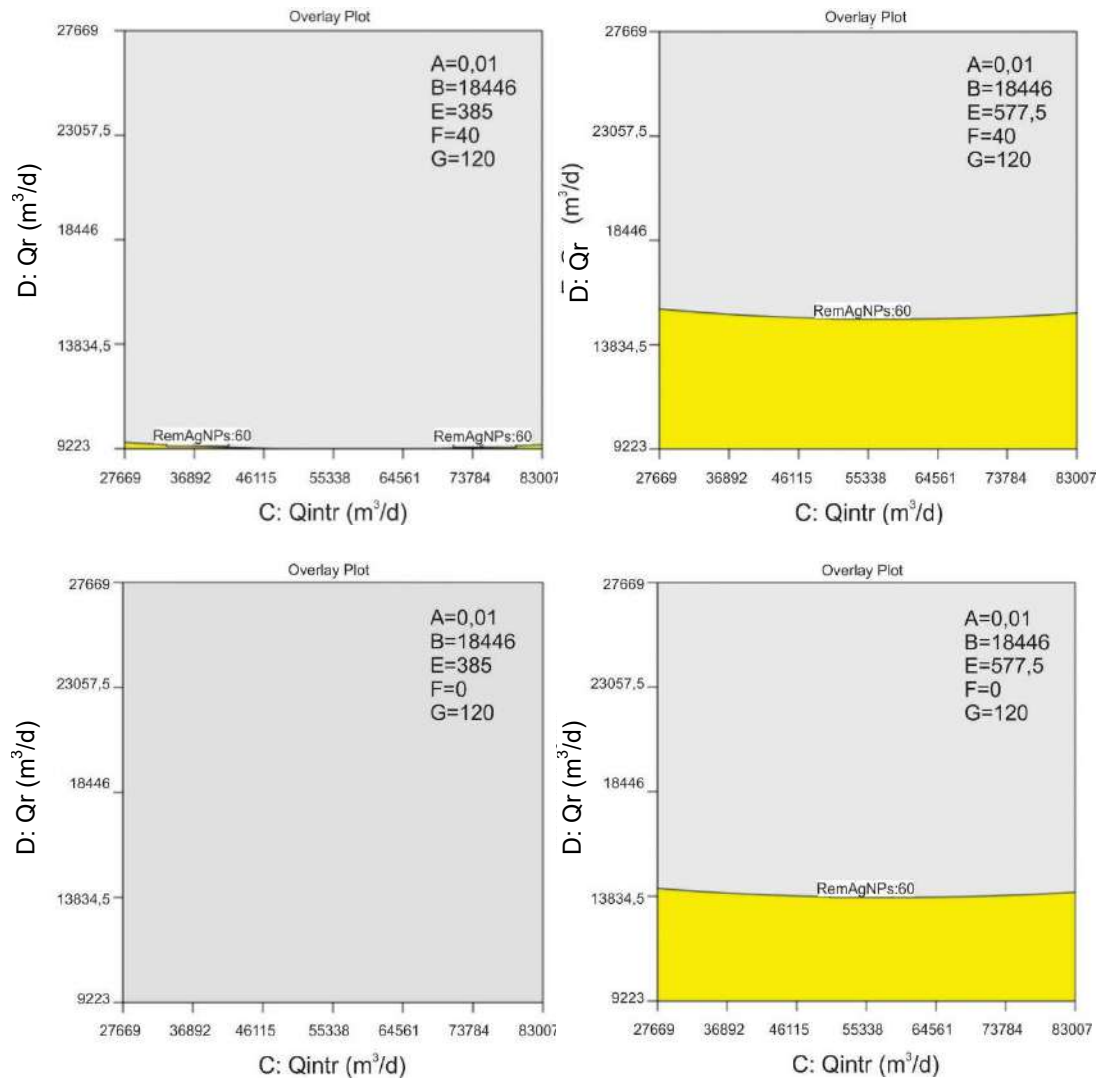
Figura A.4 - Zona óptima de las respuestas analizadas para el modelo BSM1 modificado. Escenario 1. Remoción de AgNPs 60%. Factores C: Qintr y D: Qr. A: 0,01 mgAg/L, B: 18446 m³/d, G: 120 1/d. En a) E: 385 m³/d F: 40 1/d, b) E: 577,5 m³/d F: 40 1/d, c) E: 385 m³/d F: 0 1/d, d) E: 577,5 m³/d F: 0 1/d.
