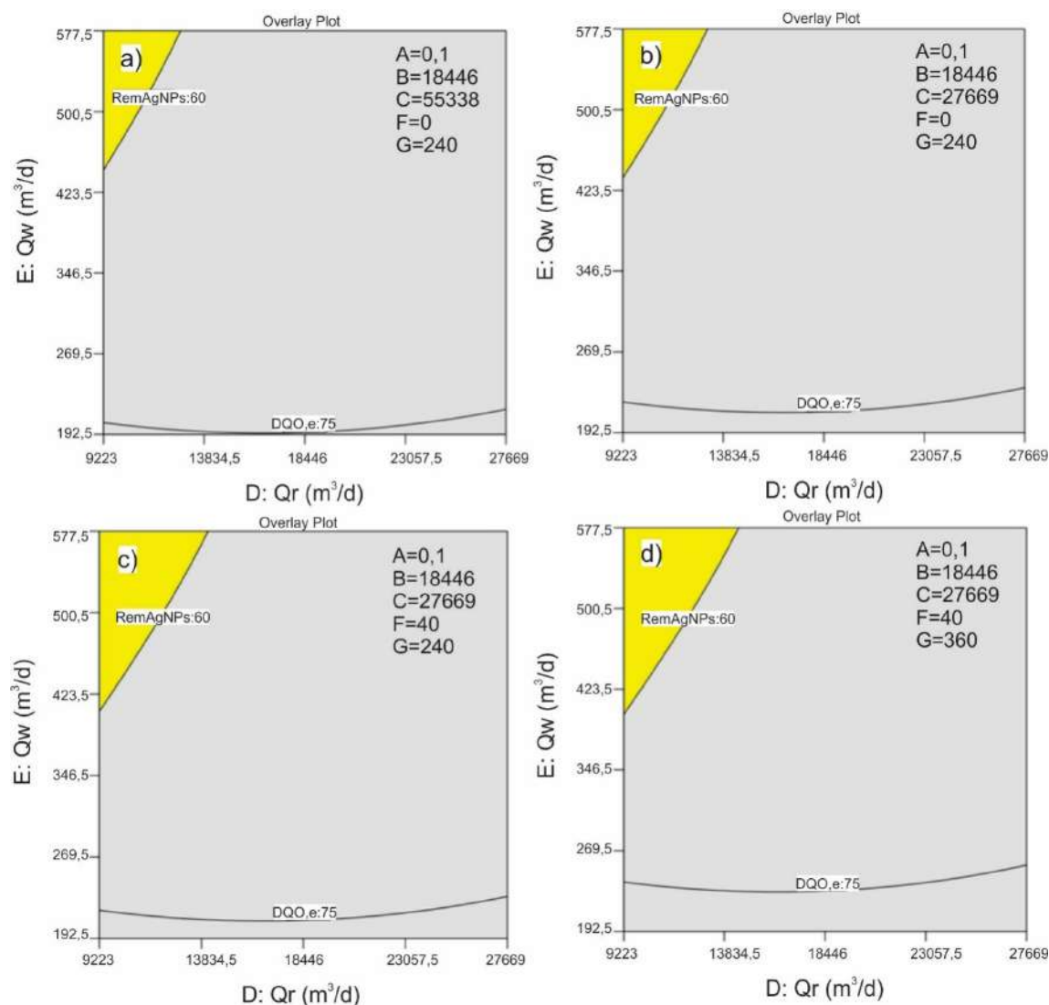
Figura 6.14 - Zona óptima de las respuestas analizadas para modelo BSM1 modificado.
