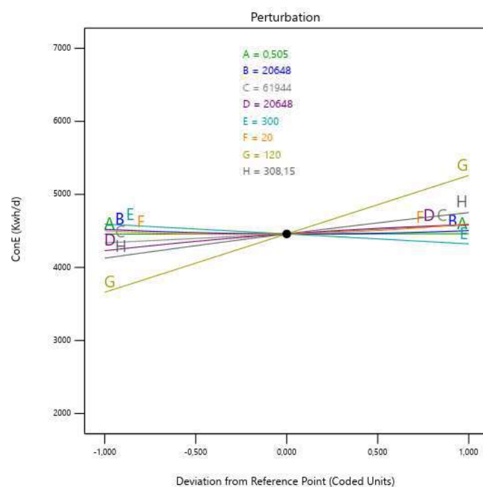
Figura 6.23 - Gráfico de perturbaciones para R2 en modelo BSM2 modificado.
