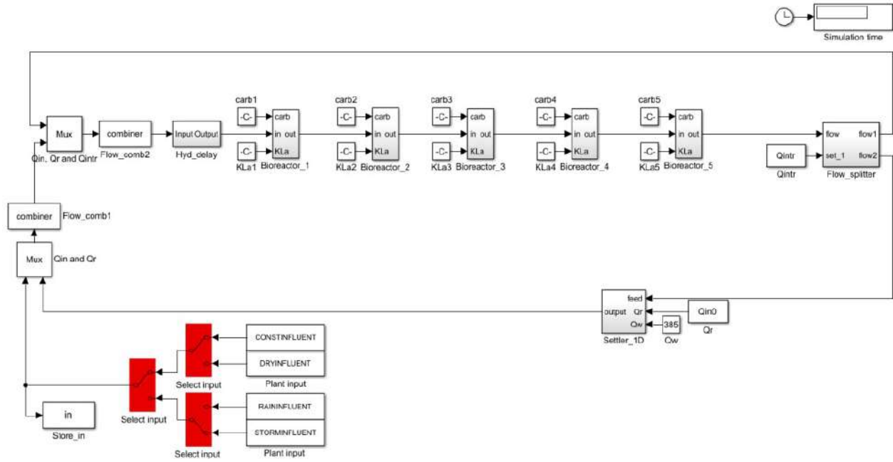
Figura 4.2 - Captura de pantalla del modelo openloop.mdl para BSM1 en MATLAB/Simulink® (Jeppson, 2011).
