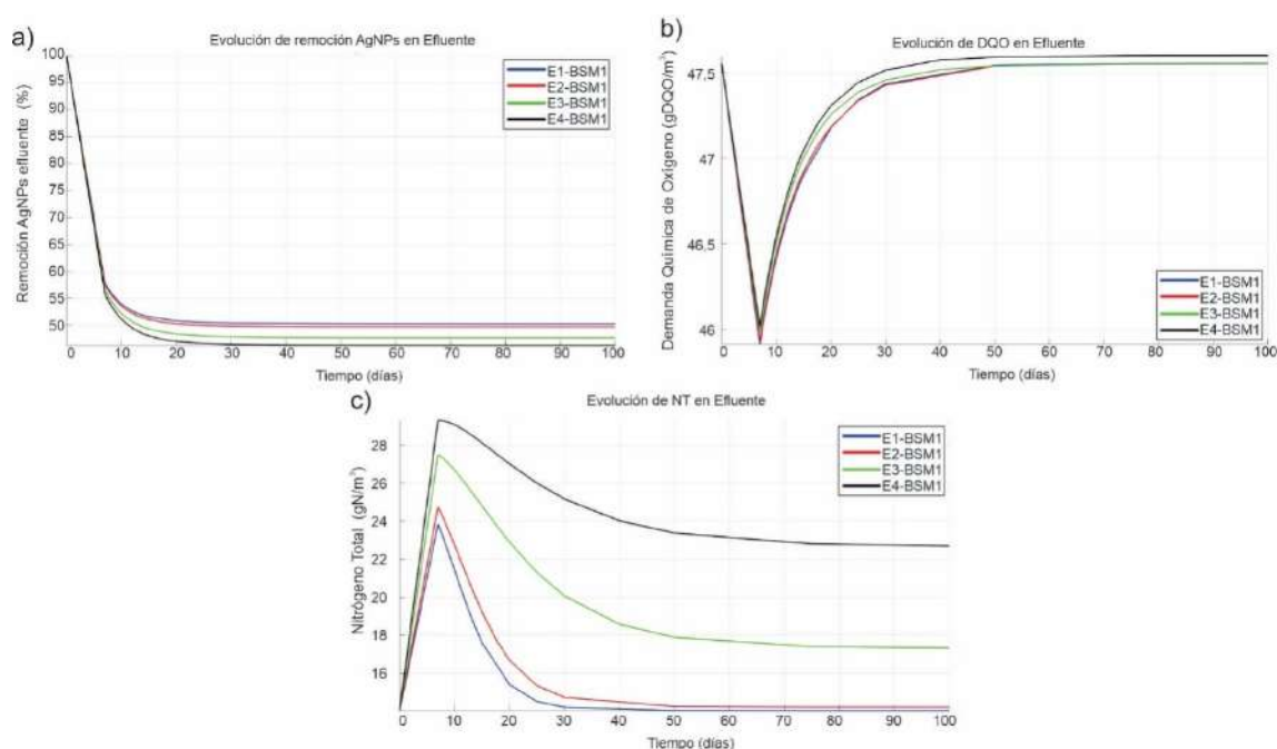
Figura 5.1 - Evolución en las salidas a) Remoción de AgNPs (%), b) DQO (mgDQO/L) y c) NT (mgN/L), durante los 100 días de simulación del modelo BSM1 modificado.
