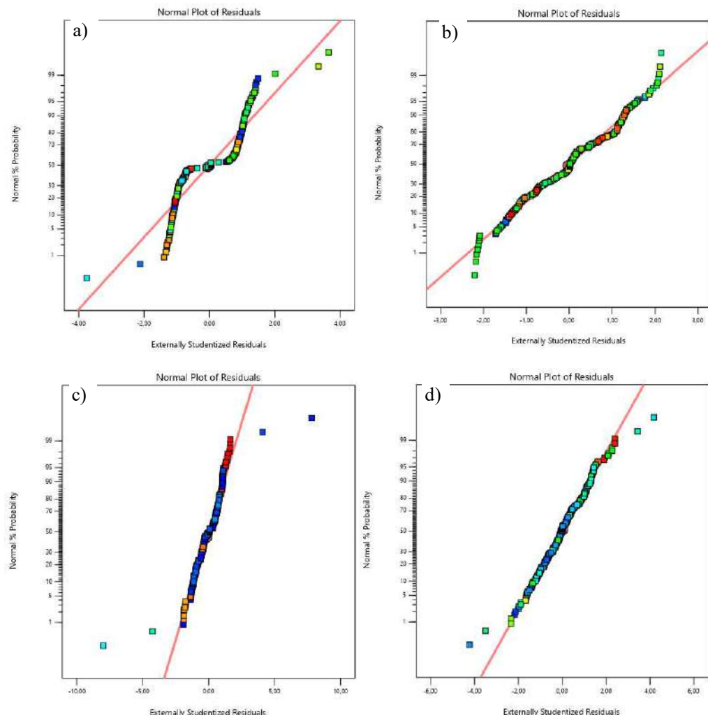
Figura 6.20 - Gráficos de residuos externamente estandarizados BSM2 modificado. a) Remoción de AgNPs, b) Consumo de Energía, c) DQO efluente, d) Nitrógeno Total efluente.
