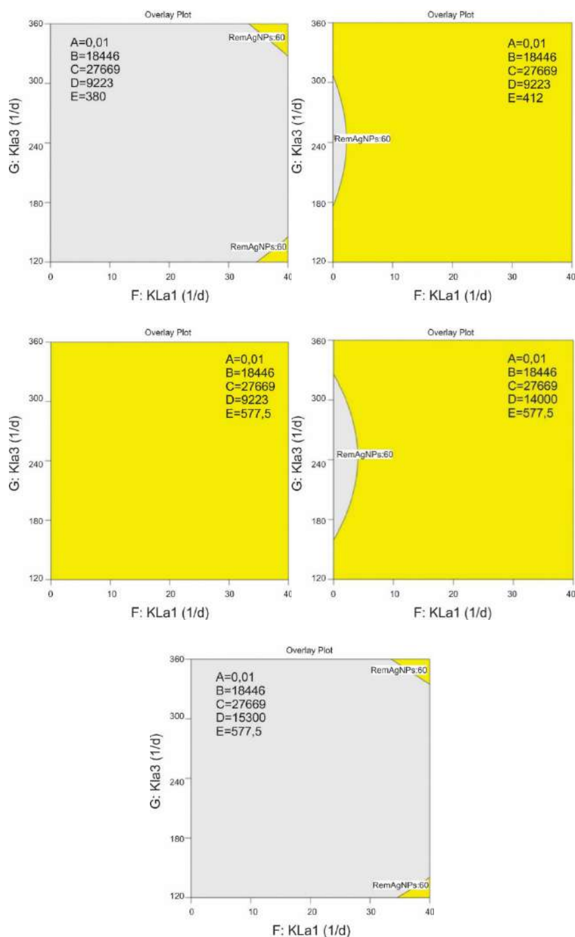
Figura A.6 - Zona óptima de las respuestas analizadas para el modelo BSM1 modificado. Escenario 1. Remoción de AgNPs 60%. Factores F: KLa1 y G: KLa3. A: 0,01 mgAg/L, B: 18846 m 3 /d, C: 27669 m 3 /d. En a) D: 9223 m 3 /d, E: 380 m 3 /d, b) D: 9223 m 3 /d, E: 412 m 3 /d, c) D: 9223 m 3 /d, E: 577,5 m 3 /d, d) D: 14000 m 3 /d, E: 577,5 m 3 /d, e) D: 15300 m 3 /d, E: 577,5 m 3 /d.
