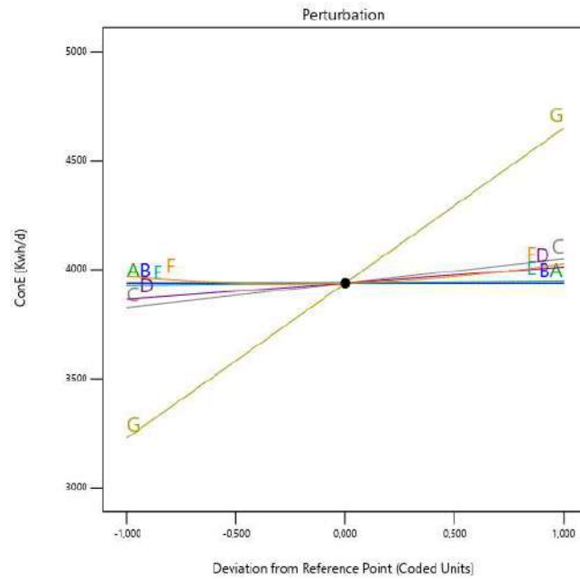
Figura 6.5 - Gráfico de perturbaciones para 'R2: ConE' en el modelo BSM1 modificado.
