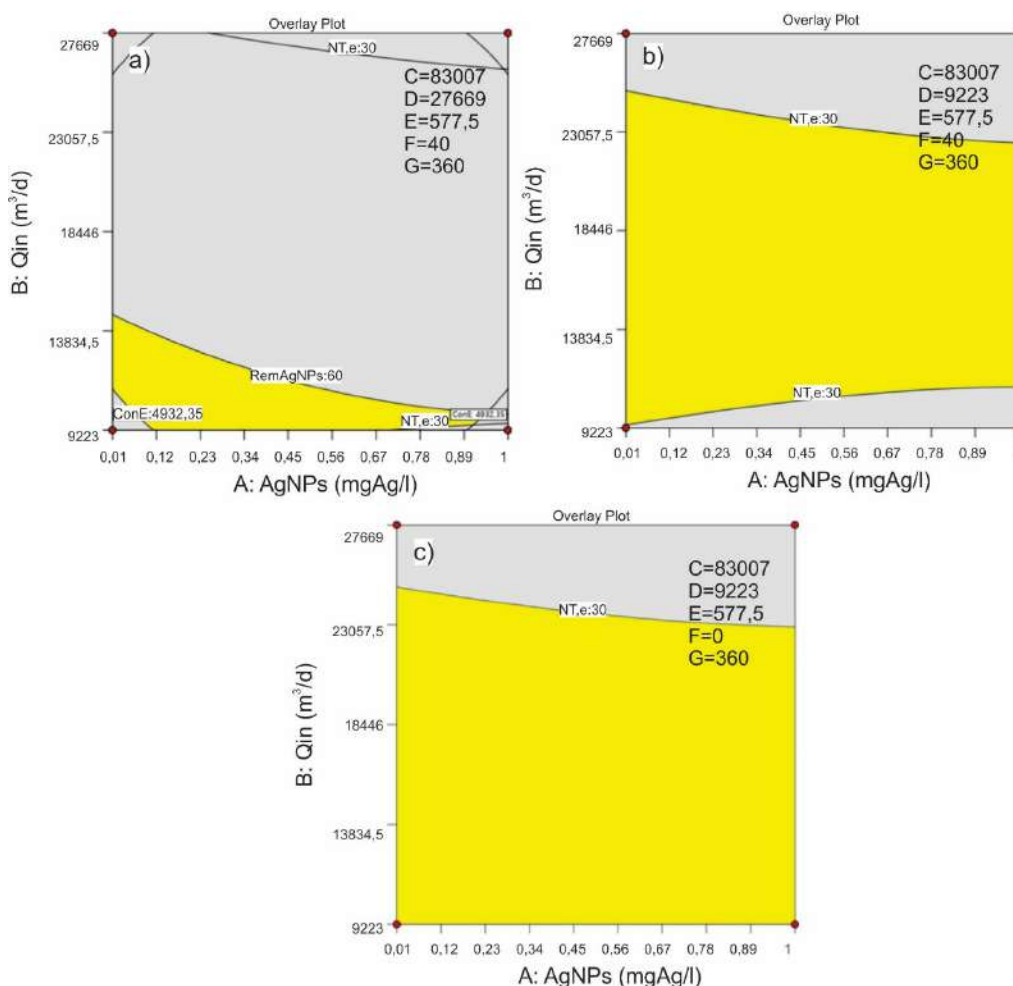
Figura 6.18 - Zona óptima de las respuestas analizadas para modelo BSM1 modificado.
