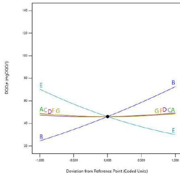
Figura 6.7- Gráfico de perturbaciones para 'R3: DQO,e' en el modelo BSM1 modificado.
