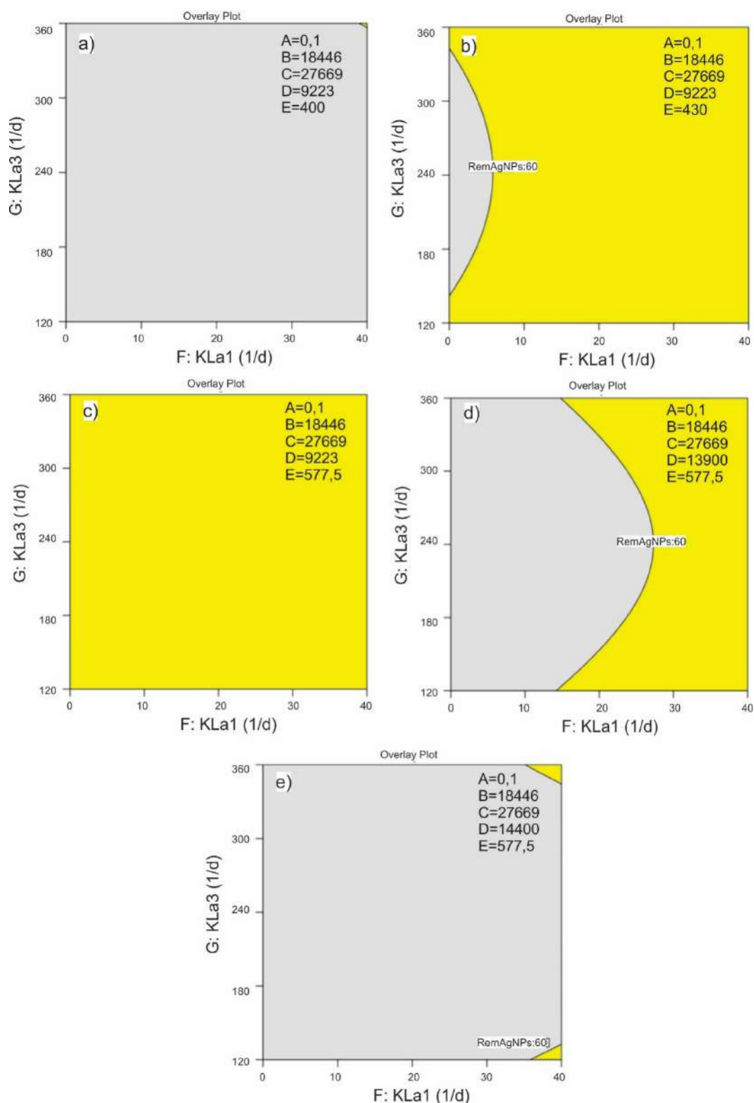
Figura 6.16 - Zona óptima de las respuestas analizadas para modelo BSM1 modificado. Remoción de AgNPs 60%. Factores F: K_{La1} (1/d), G: K_{La3} (1/d). A: 0,1 mgAg/L, B: 18446 m^3/d , C: 27669 m^3/d . En a) D: 9223 m^3/d , E: 400 m^3/d , b) D: 9223 m^3/d , E: 430 m^3/d , c) D: 9223 m^3/d , E: 577,5 m^3/d , d) D: 13900 m^3/d , E: 577,5 m^3/d , e) D: 14400 m^3/d , E: 577,5 m^3/d .
