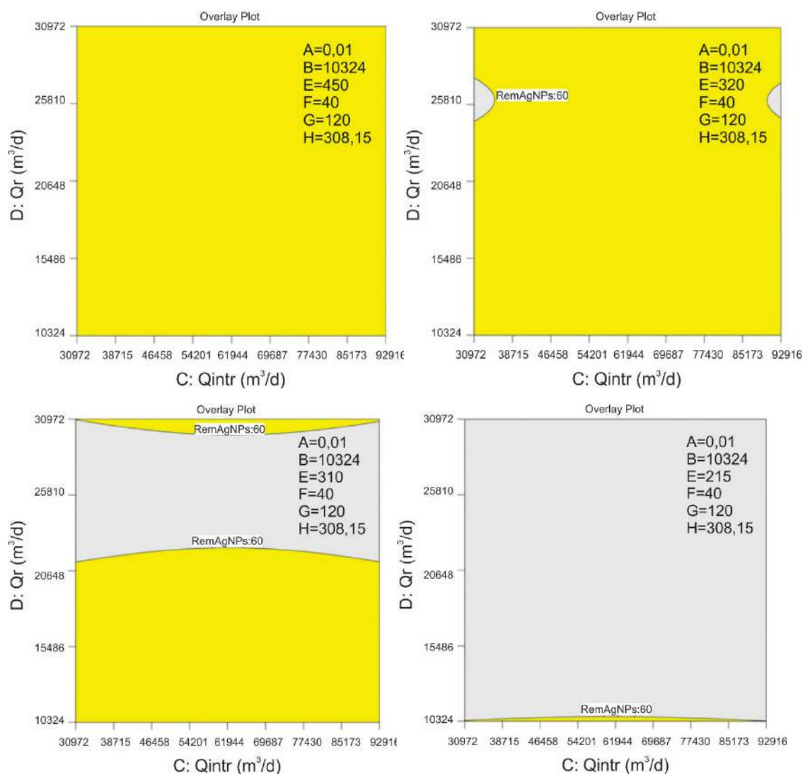
Figura A.22 - Zona óptima de las respuestas analizadas para el modelo BSM2 modificado. Escenario 1. Remoción de AgNPs 60%. Factores C: Qintr y D: Qr. A: 0,01mgAg/L, B: 10324 m³/d, F: 40 1/d, G: 120 1/d, H: 308,15 K. En a) E: 450 m³/d, b) E: 320 m³/d, c) E: 310 m³/d, d) E: 215 m³/d.
