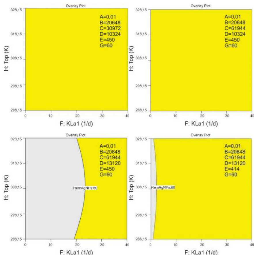
Figura A.24 - Zona óptima de las respuestas analizadas para el modelo BSM2 modificado. Escenario 1. Remoción de AgNPs 60%. Factores F: KLa1 y H: Top. A: 0,01 mgAg/L, B: 20648 m³/d, G: 60 1/d. En a) C: 30972 m³/d, D: 10324 m³/d, E: 450 m³/d, b) C: 61944 m³/d, D: 10324 m³/d, E: 450 m³/d, c) C: 61944 m³/d, D: 13120 m³/d, E: 450 m³/d, d) C: 61944 m³/d, D: 13120 m³/d, E: 414 m³/d.
