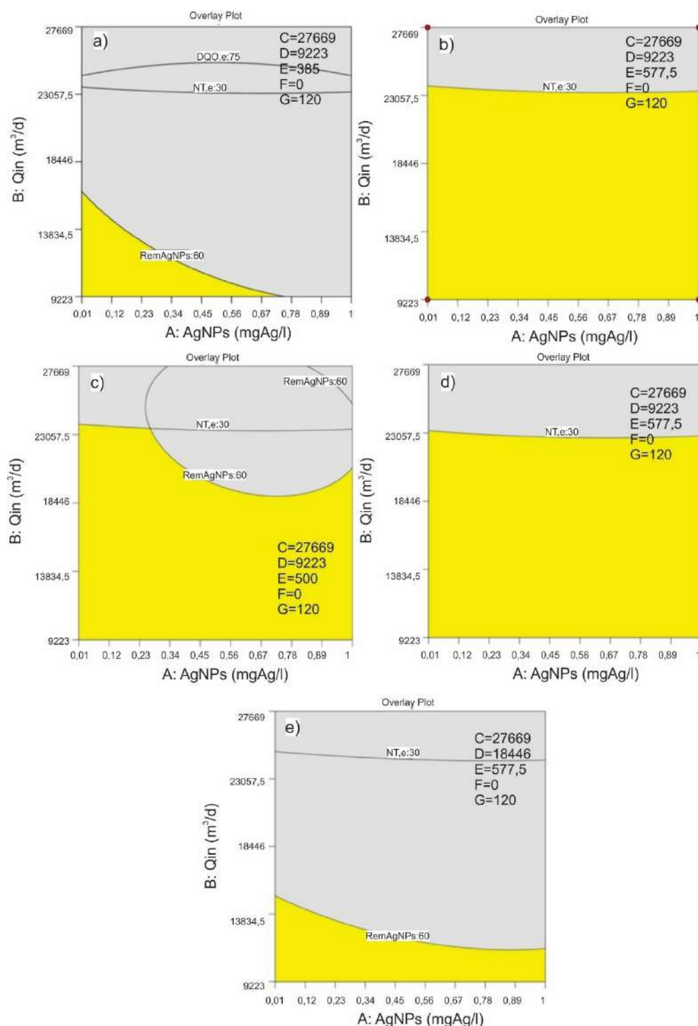
Figura 6.17 - Zona óptima de las respuestas analizadas para modelo BSM1 modificado. Remoción de AgNPs 60%. Factores A: AgNPs y B: Qin. F: 0 l/d, G: 120 l/d. En a) C: 27669 m³/d, D: 9223 m³/d, E: 385 m³/d, b) C: 27669 m³/d, D: 9223 m³/d, E: 577,5 m³/d, c) C: 27669 m³/d, D: 9223 m³/d, E: 500 m³/d, d) C: 55338 m³/d, D: 9223 m³/d, E: 577,5 m³/d, e) C: 27669 m³/d, D: 18446 m³/d, E: 577,5 m³/d.
