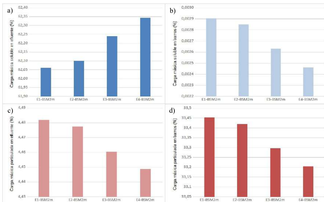
Figura 5.7 - Porcentaje de carga másica de especies de plata en efluente y barros para cuatro escenarios de concentración inicial de AgNPs para el modelo BSM2 modificado. a) porcentaje de especies solubles en efluente, b) porcentaje de especies solubles en barros, c) porcentaje de especies particuladas en efluentes, d) porcentaje de especies particuladas en barros.
