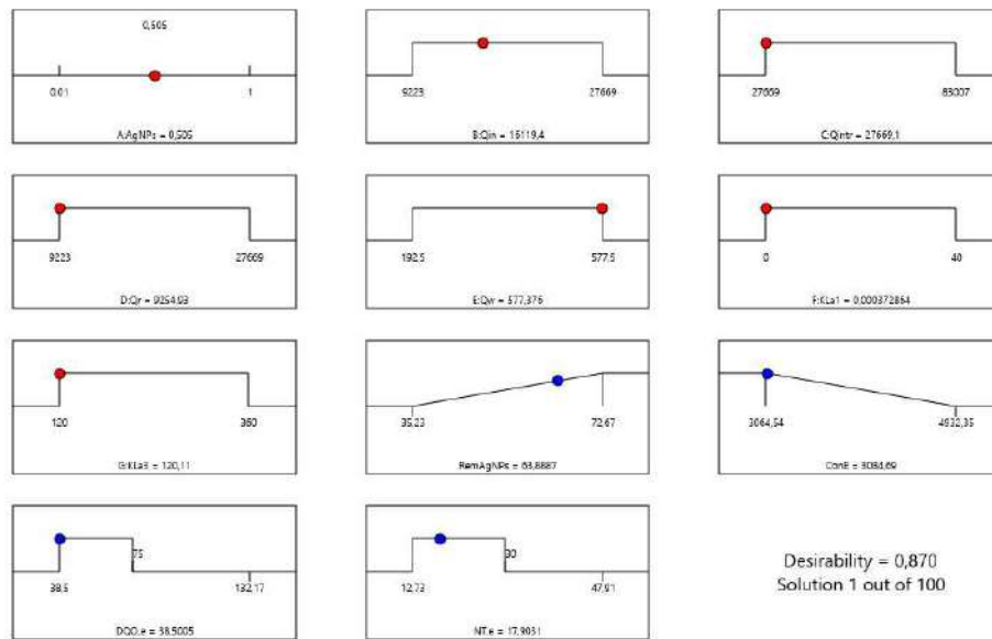
Figura A.7 - Optimización numérica para el Escenario 3-A., para el modelo BSM1 modificado. AgNPS: 0,505mgAg/L, Qin libre. Deseabilidad: 0,870.
