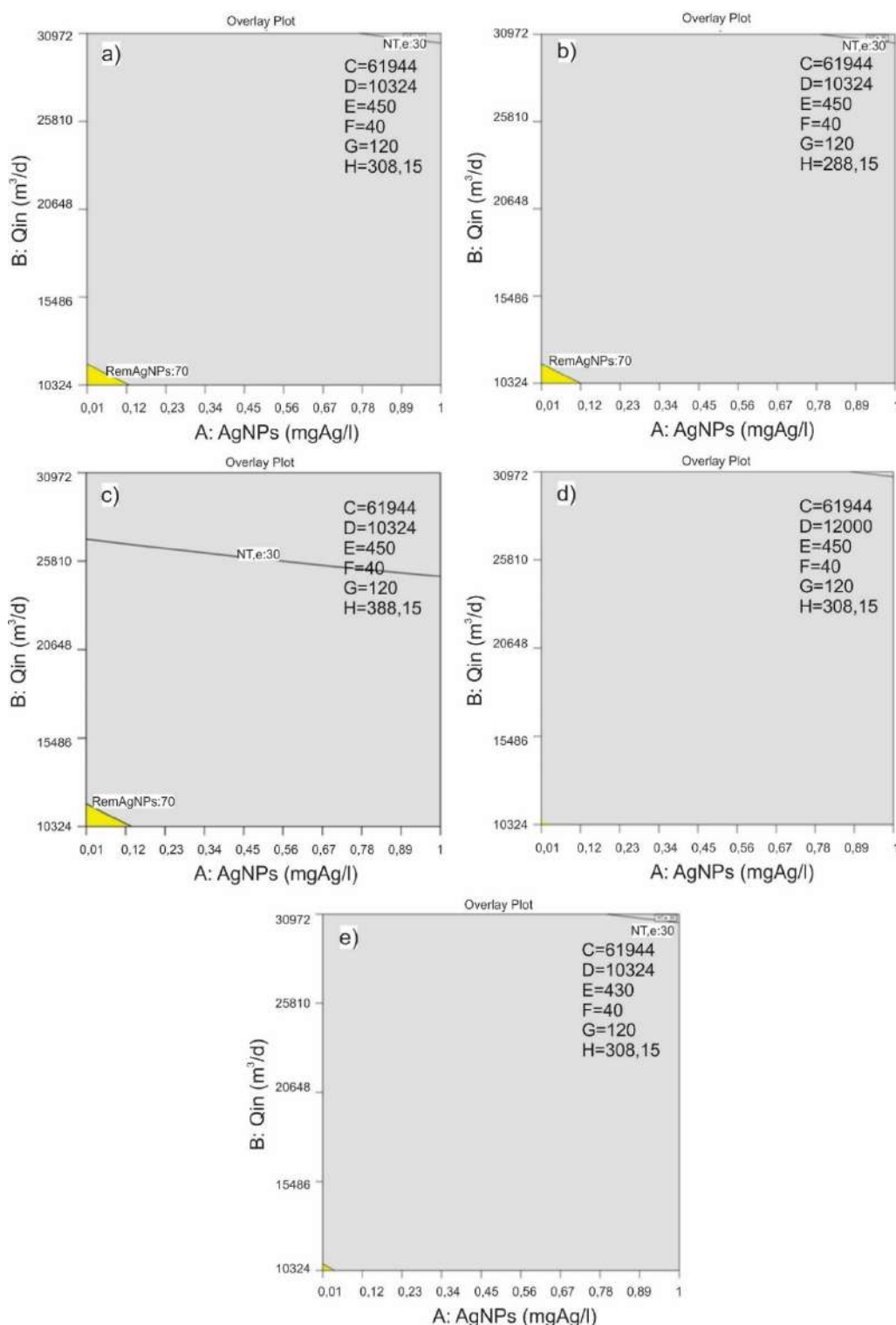
Figura 6.37 - Zona óptima de las respuestas analizadas para el modelo BSM2 modificado. Remoción de AgNPs 70%. Factores A: AgNPs y B: Qin. C: 61944 m³/d, F: 40 l/d, G: 120 l/d. En a) D: 10324 m³/d, E: 450 m³/d, H: 308,15 K, b) D: 10324 m³/d, E: 450 m³/d, H: 288,15 K, c) D: 10324 m³/d, E: 450 m³/d, H: 388,15 K, d) D: 12000 m³/d, E: 450 m³/d, H: 308,15 K, e) D: 10324 m³/d, E: 430 m³/d, H: 308,15 K.
