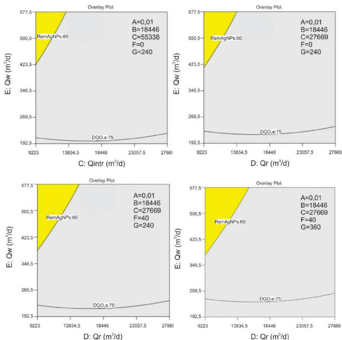
Figura A.5 - Zona óptima de las respuestas analizadas para el modelo BSM1 modificado. Escenario 1. Remoción de AgNPs 60%. Factores D: Qr y E: Qw. A: 0,01 mgAg/L, B: 18846 m³/d. En a) C: 55338 m³/d, F: 0 l/d, G: 240 l/d, b) C: 27669 m³/d, F: 0 l/d, G: 240 l/d, c) C: 27669 m³/d, F: 40 l/d, G: 240 l/d, d) C: 27669 m³/d, F: 40 l/d, G: 360 l/d,
