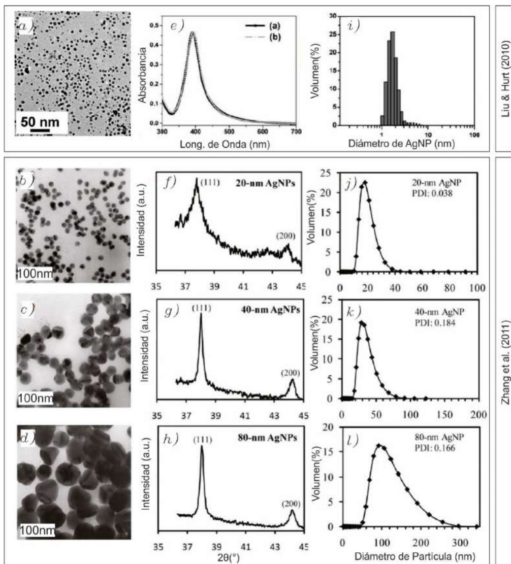
Figura 3.2 - Morfología, distribución de tamaños de AgNPs, espectros de absorción de UV-vis y patrón de difracción de rayos-X. Adaptado de Liu & Hurt (2010) y Zhang et al. (2011). a), b), c), d) imágenes TEM de AgNPs de 2, 20, 40 y 80 nm, respectivamente; e) absorción de espectro UV-vis de AgNPs suspendidas en agua destilada e)(a) recién realizada la suspensión, e)(b) luego de 5 meses de almacenada a 4°C, el pico de absorbancia a 390 nm permanece invariable, indicando la estabilidad del tamaño y la forma de las AgNPs en la suspensión. f), g), h), patrón de difracción de rayos X; i), j), k), l) distribución de tamaño in situ por DLS.
