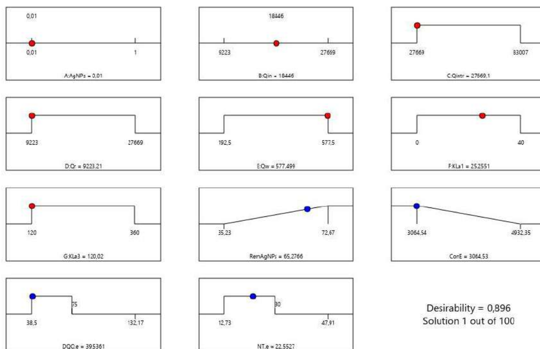
Figura A.2 - Optimización numérica para el Escenario 1-B., para el modelo BSM1 modificado. AgNPs 0,01 mg/L, Qin: 18446 m 3 /d. Deseabilidad: 0,896.
