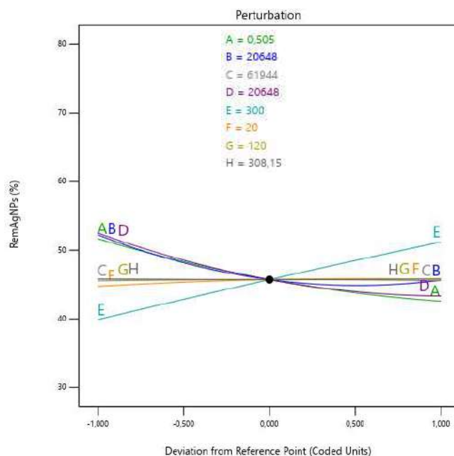
Figura 6.21 - Gráfico de perturbaciones para R1 en modelo BSM2 modificado.
