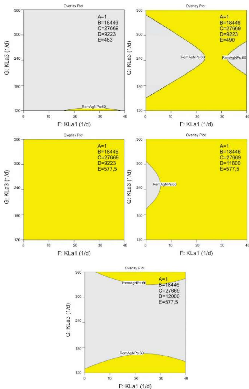
Figura A.18 - Zona óptima de las respuestas analizadas para el modelo BSM2 modificado.
