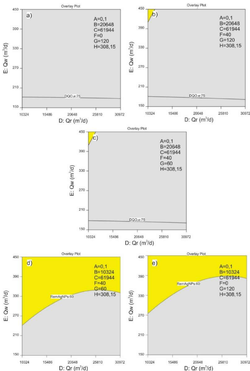
Figura 6.35 - Zona óptima de las respuestas analizadas para el modelo BSM2 modificado. Remoción de AgNPs 60%. Factores D: Qr y E: Qw. A: 0,1 mgAg/L, C: 61944 m³/d, H: 308,15 K. En a) B: 20648 m³/d, F: 0 1/d, G: 120 1/d, b) B: 20648 m³/d, F: 40 1/d, G: 120 1/d, c) B: 20648 m³/d, F: 40 1/d, G: 60 1/d, d) B: 10324 m³/d, F: 40 1/d, G: 60 1/d, e) B: 10324 m³/d, F: 0 1/d, G: 120 1/d.
