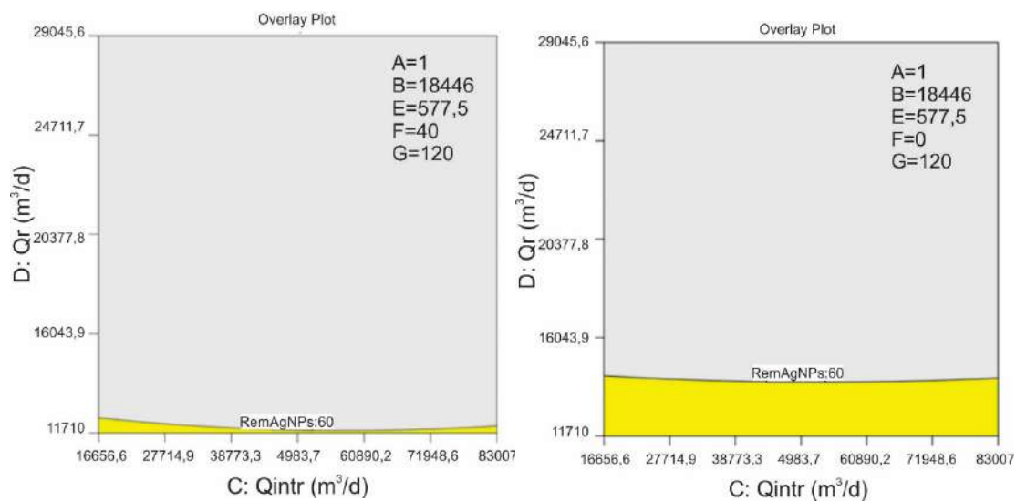
Figura A.15 - Zona óptima de las respuestas analizadas para el modelo BSM1 modificado. Escenario 4. Remoción de AgNPs 60%. Factores C: Qintr y D: Qr. A: 1mgAg/L, B: 18446 m³/d, E: 577,5 m³/d, G: 120 l/d. En a) F: 40 l/d, b) F: 0 l/d.
