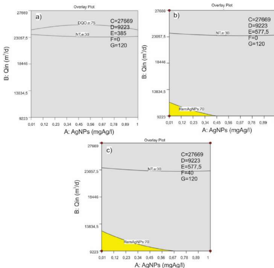
Figura 6.19 - Zona óptima de las respuestas analizadas para modelo BSM1 modificado. Remoción de AgNPs 70%. Factores A: AgNPs y B: Qin. C: 27669m 3 /d, D: 9223m 3 /d, G: 120 1/d. En a) E: 385 m 3 /d, F: 0 1/d, b) E: 577,5 m 3 /d, F: 0 1/d, c) E: 577,5 m 3 /d, F: 40 1/d.
