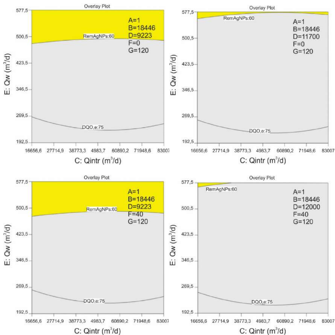
Figura A.16 - Zona óptima de las respuestas analizadas para el modelo BSM1 modificado. Escenario 4. Remoción de AgNPs 60%. Factores C: Qintr y E: Qw. A: 1 mgAg/L, B: 18446 m³/d, G: 120 1/d. En a) D: 9223 m³/d, F: 0 1/d, b) D: 11700 m³/d, F: 0 1/d, c) D: 9223 m³/d, F: 40 1/d, d) D: 12000 m³/d, F: 40 1/d.
