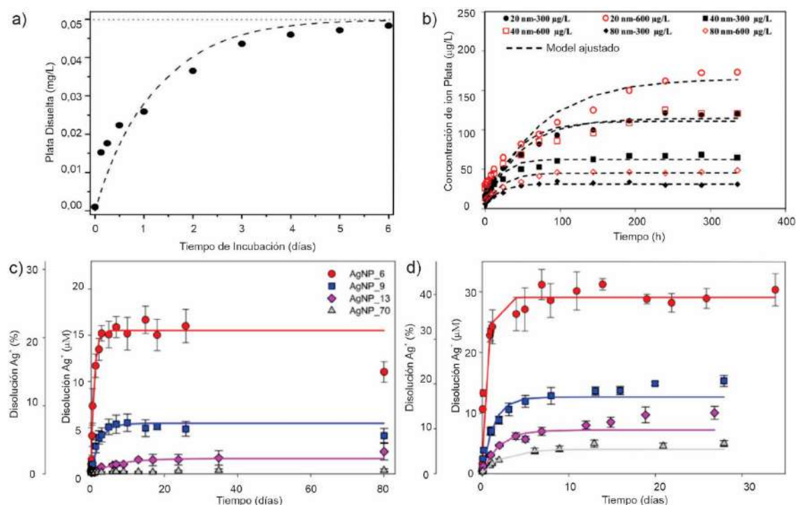
Figura 3.4 - Cinética de disolución de AgNPs o liberación de iones Ag^+ . a) Liu & Hurt (2010), ajuste de cinética empírica para disolución de plata, suspensión de 0,05 mg/L de AgNPs (9,1 mg/L de O_2 disuelto, agua destilada a 20°C, sin luz); b) Zhang et al. (2011), ajuste de cinética de liberación de Ag^+ en un medio Hoagland a un cuarto de concentración; c) y d) Peretyazkho et al. (2014), Ag^+ disuelto en µM y % ( [Ag^+]/[Ag]_{total} \times 100\% ), para una suspensión de 74 µM de AgNPs, en c) agua, d) ácido acético 0,05 M.
