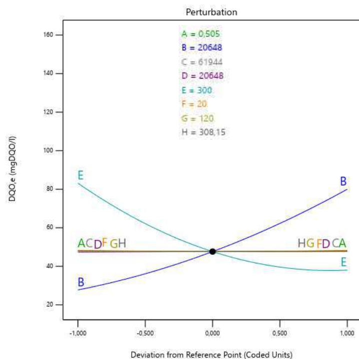
Figura 6.25 - Gráfico de perturbaciones para R3: DQO, en el modelo BSM2 modificado.
