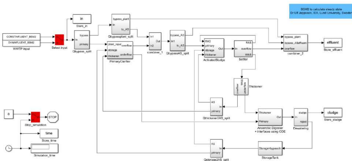
Figura 4.4 - Captura de pantalla del modelo bsm2_ss.mdl para BSM2 en MATLAB/Simulink® (Jeppson, 2011).
