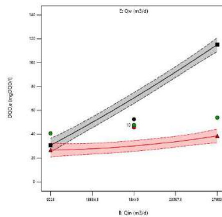
Figura 6.8 - Gráficos de las interacciones más significativas entre los factores BE, para la respuesta 'R3: DQO,e' en el modelo BSM1 modificado.
