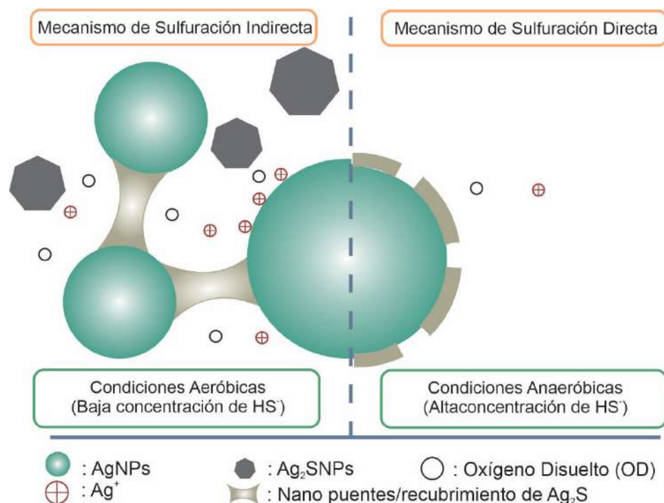
Figura 3.8 – Mecanismos de sulfuración indirecta y directa para las AgNPs. Condiciones, especies involucradas y formas en las que se puede encontrar el \text{Ag}_2\text{S} formado. Adaptado de Zhang et al. (2018).
