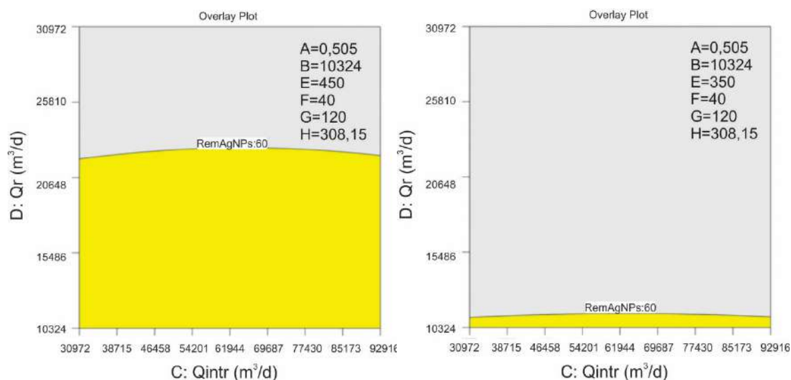
Figura A.28 - Zona óptima de las respuestas analizadas para el modelo BSM2 modificado. Escenario 3. Remoción de AgNPs 60%. Factores D: Qr y E: Qw. A: 0,505mgAg/L, B: 10324 m³/d, F: 40 l/d, G: 120 l/d, H: 308,15 K. En a) E: 450 m³/d, b) E: 350 m³/d.
