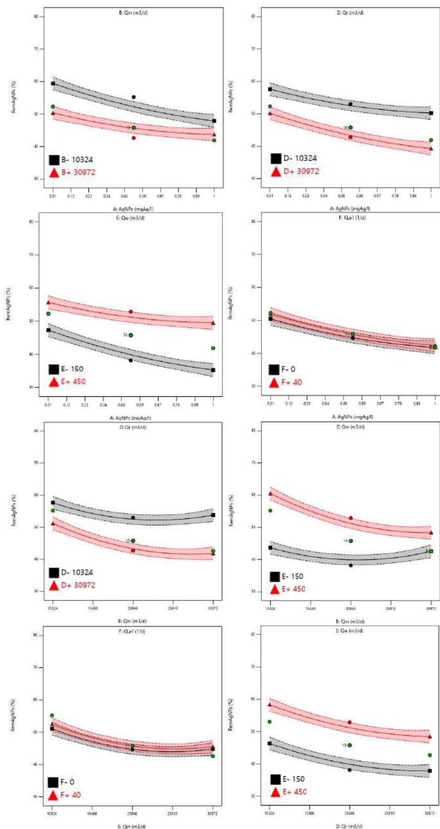
Figura 6.22 - Gráficos de las interacciones más significativas entre los factores: a) AB, b) AD, c) AE, d) AF, e) BD, f) BE, g) BF y h) DE, para la respuesta 'R1: Remoción de AgNPs' en el modelo BSM2 modificado.
