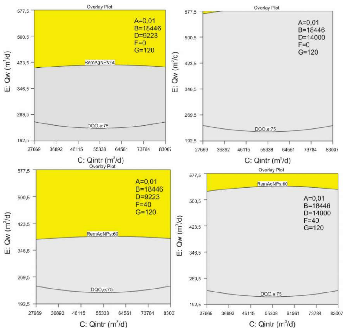
Figura A.3 - Zona óptima de las respuestas analizadas para el modelo BSM1 modificado. Escenario 1. Remoción de AgNPs 60%. Factores C: Qintr y E: Qw. A: 0,01 mgAg/L, B: 18446 m³/d, G: 120 1/d. En a) D: 9223 m³/d, F: 0 1/d, b) D: 14000 m³/d, F: 0 1/d c) D: 9223 m³/d, F: 40 1/d, d) D: 14000 m³/d, F: 40 1/d.
