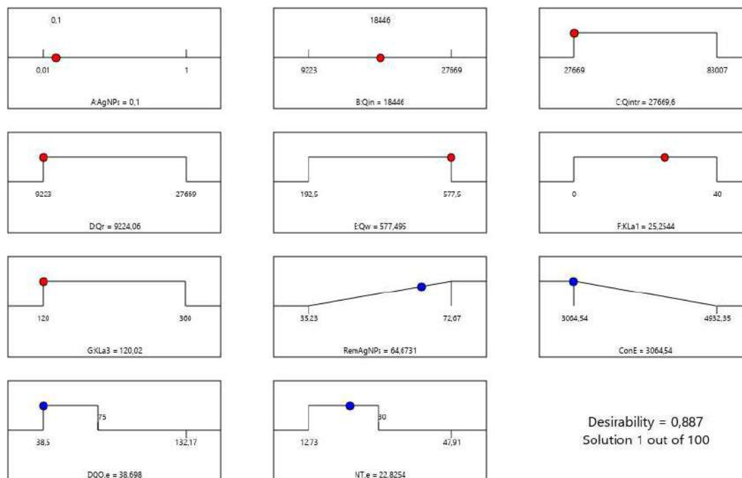
Figura 6.12 - Optimización numérica de la función de deseabilidad utilizando RSM para el Escenario 2-B, BSM1 modificado. AgNPS: 0,1 mgAg/L, Qin: 18446 m 3 /d. Deseabilidad: 0,887.
