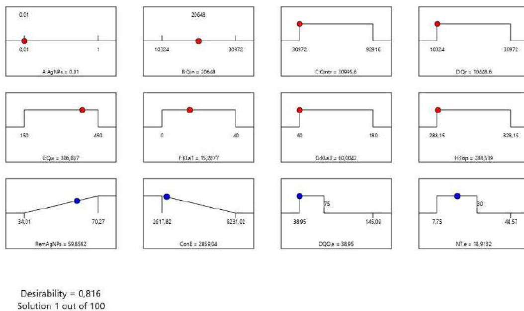
Figura A.20 - Optimización numérica para el Escenario 1-A, para el modelo BSM2 modificado. AgNPS: 0,01 mgAg/L, Qin 20648 m 3 /d. Deseabilidad: 0,816.
