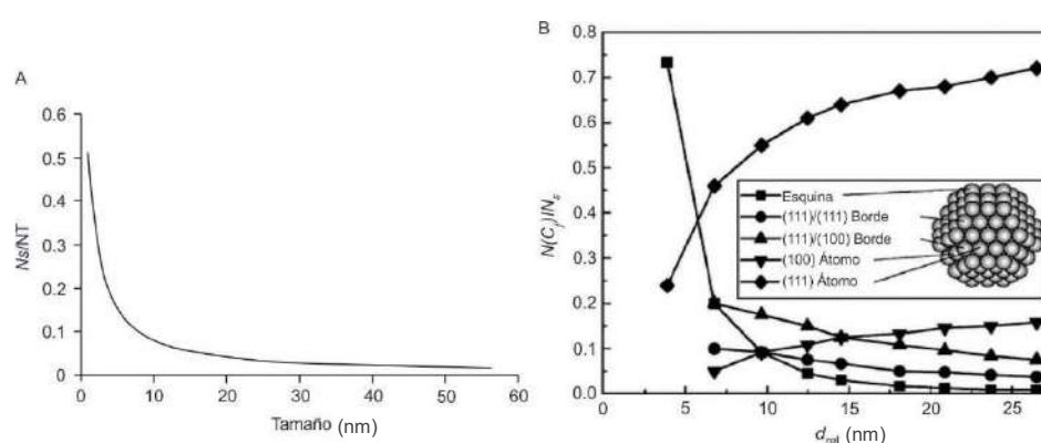
Figura 2.3 - Relación átomos de superficie y átomos totales para distintos tamaños de nanopartículas. (A) Reducción exponencial del área superficial específica en la nanoescala; (B) distribución de átomos en distintos sitios de superficie en una nanopartícula. Adaptado de Baalousha et al. (2014).
