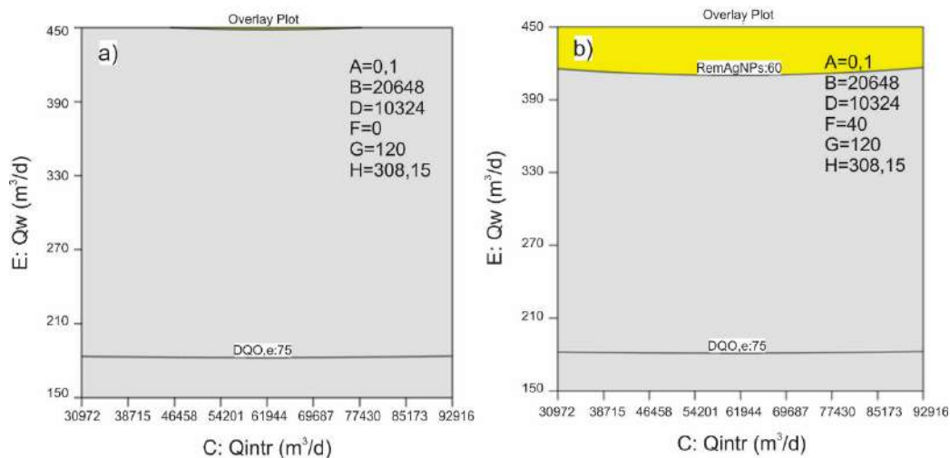
Figura 6.33 - Zona óptima de las respuestas analizadas para el modelo BSM2 modificado. Remoción de AgNPs 60%. Factores C: Qintr y E: Qw. A: 0,1 mgAg/L, B: 20648 m 3 /d, D: 10324 m 3 /d, G: 120 1/d H: 308,15 K. En a) F: 0 1/d, b) F: 40 1/d.
