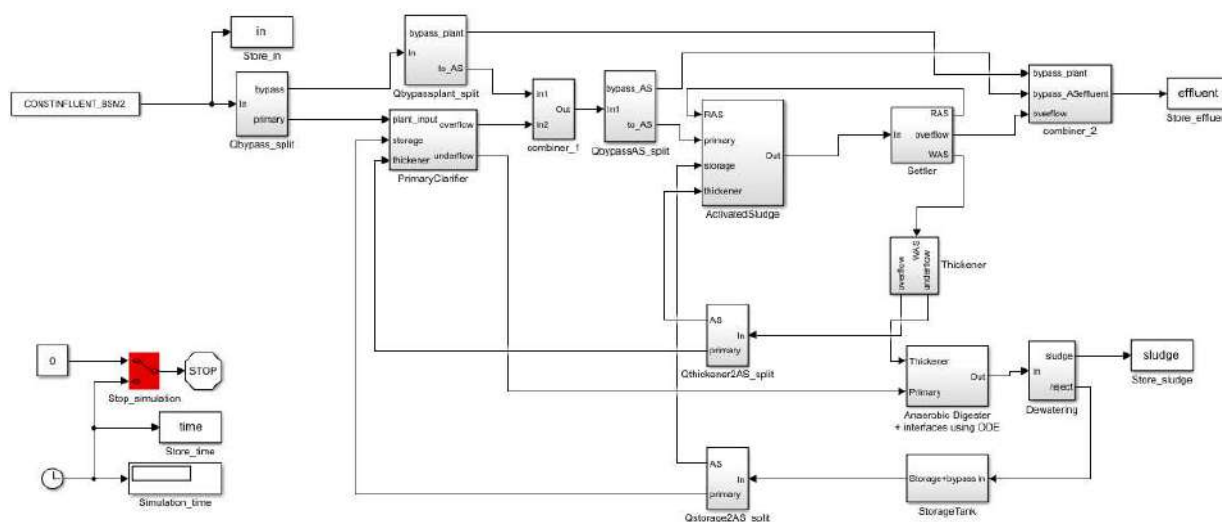
Figura 4.6 - Vista de captura de pantalla del modelo BSM2 modificado en MATLAB/Simulink®.
