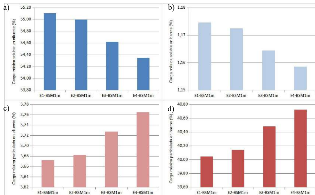
Figura 5.3 - Porcentaje de carga másica de especies de plata en efluente y barros para cuatro escenarios en el modelo BSM1 modificado. Porcentajes de especies solubles a) en efluente, b) en barros, y especies particuladas c) en efluentes y d) en barros.
