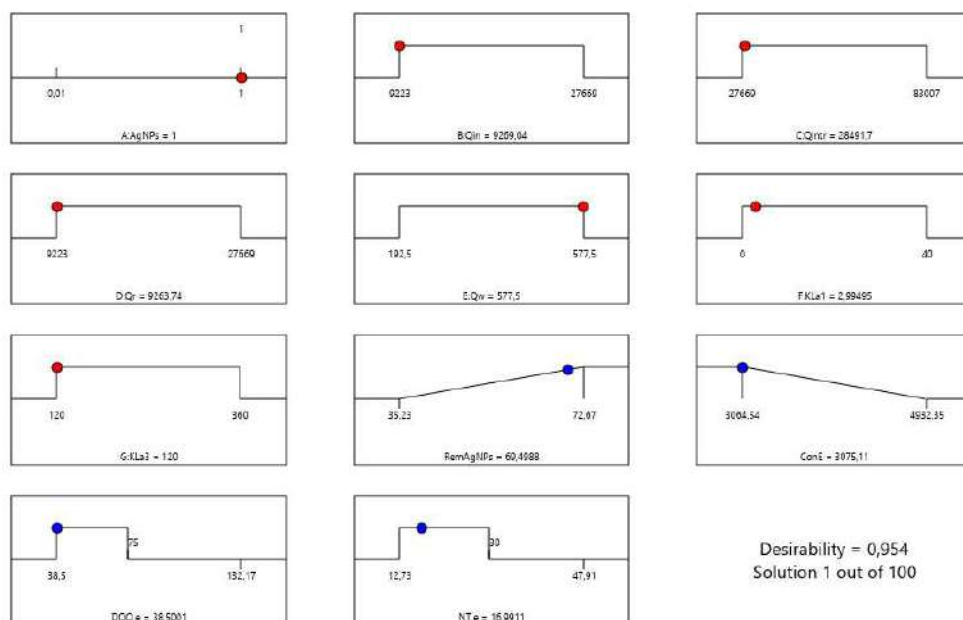
Figura A.13 - Optimización numérica de la función de deseabilidad utilizando RSM para el Escenario 4-A, BSM1 modificado. AgNPS: 1 mgAg/L, Qin: libre.
