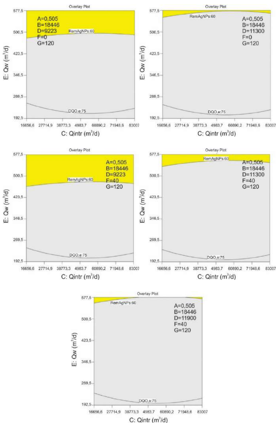
Figura A.10 - Zona óptima de las respuestas analizadas para el modelo BSM1 modificado. Escenario 3. Remoción de AgNPs 60%. Factores C: Qintr y E: Qw. A: 0,505mgAg/L, B: 18446 m³/d, G: 120 1/d. En a) D: 9223 m³/d, F: 0 1/d, b) D: 11300 m³/d, F: 0 1/d, c) D: 9223 m³/d, F: 40 1/d, d) D: 11300 m³/d, F: 40 1/d, e) D: 11900 m³/d, F: 40 1/d.
