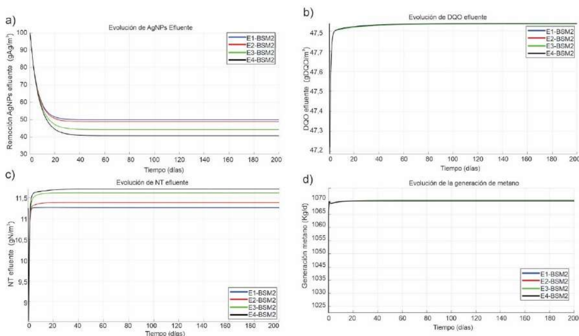
Figura 5.4 - Evolución en las salidas durante los 200 días de corrida del modelo BSM2 modificado de: a) Remoción de AgNPs, b) DQO efluente, c) NT efluente y d) Generación de metano.
