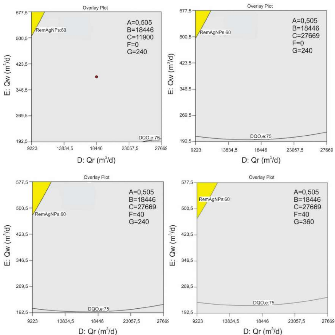
Figura A.11 - Zona óptima de las respuestas analizadas para el modelo BSM1 modificado. Escenario 3. Remoción de AgNPs 60%. Factores D: Qr y E: Qw. A: 0,505mgAg/L, B: 18446 m³/d. En a) C: 11900 m³/d, F: 0 l/d, G: 240 l/d, b) C: 27669 m³/d, F: 0 l/d, G: 240 l/d, c) C: 27669 m³/d, F: 40 l/d, G: 240 l/d, d) C: 27669 m³/d, F: 40 l/d, G: 360 l/d.
