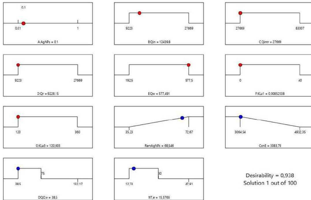
Figura 6.11 - Optimización numérica de la función de deseabilidad utilizando RSM para el Escenario 2-A, BSM1 modificado. AgNPS: 0,1 mgAg/L, Qin libre. Deseabilidad: 0,938.
