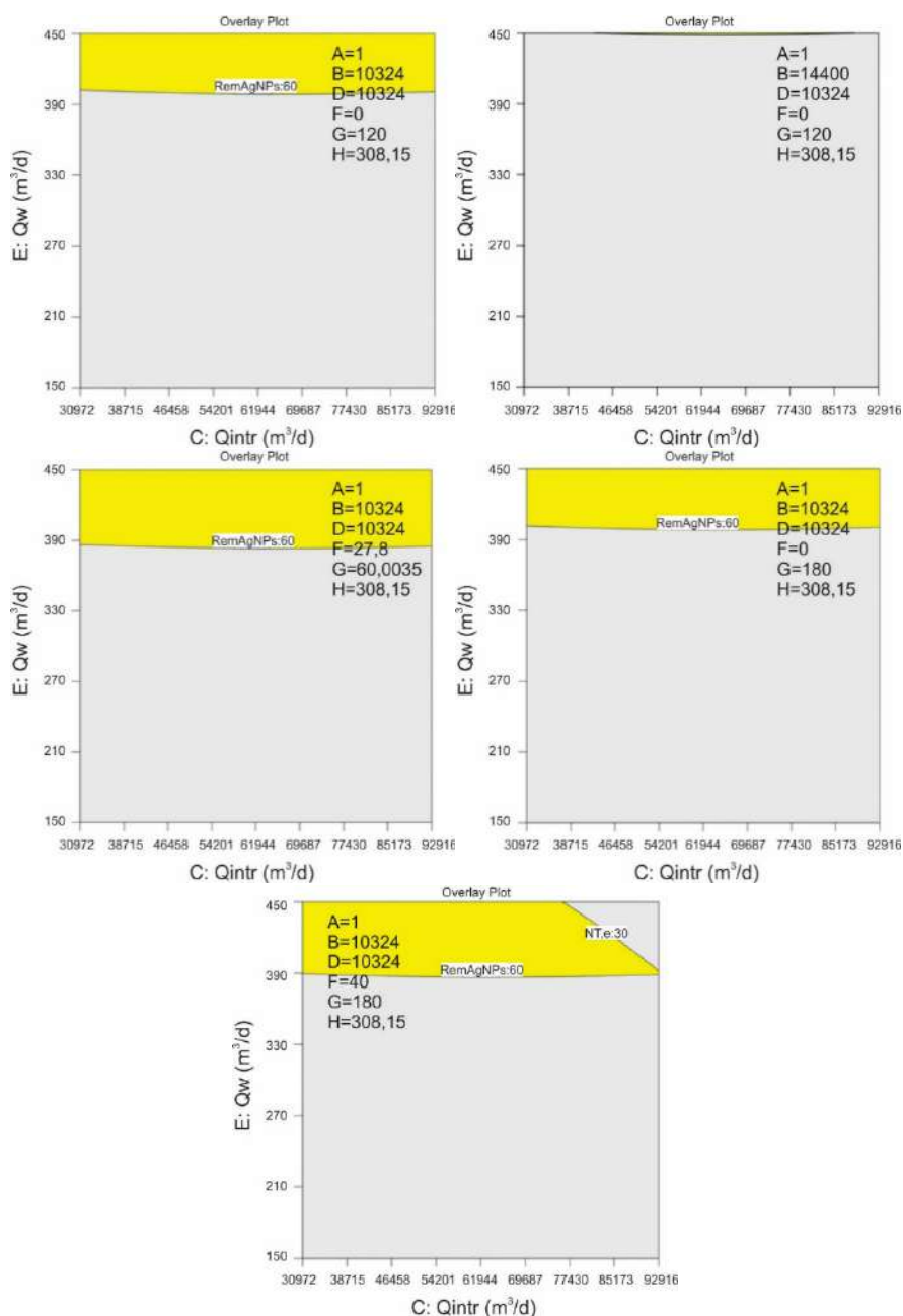
Figura A.35 - Zona óptima de las respuestas analizadas para el modelo BSM2 modificado. Escenario 4. Remoción de AgNPs 60%. Factores C: Qintr y E: Qw. A: 1 mgAg/L, D: 10324 m³/d, H: 308,15 K. En a) B: 10324 m³/d, F: 0 1/d, G: 120 1/d, b) B: 14400 m³/d, F: 0 1/d, G: 120 1/d, c) B: 10324 m³/d, F: 27,8 1/d, G: 60,0035 1/d, d) B: 10324 m³/d, F: 0 1/d, G: 180 1/d, e) B: 10324 m³/d, F: 40 1/d, G: 180 1/d.
