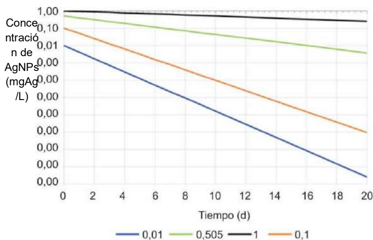
Figura 5.8 - Concentración de AgNPs en función del tiempo para las concentraciones de los cuatro escenarios (0,01; 0,1; 0,505; 1 mgAg/L de AgNPs). Eje vertical en escala logarítmica.
