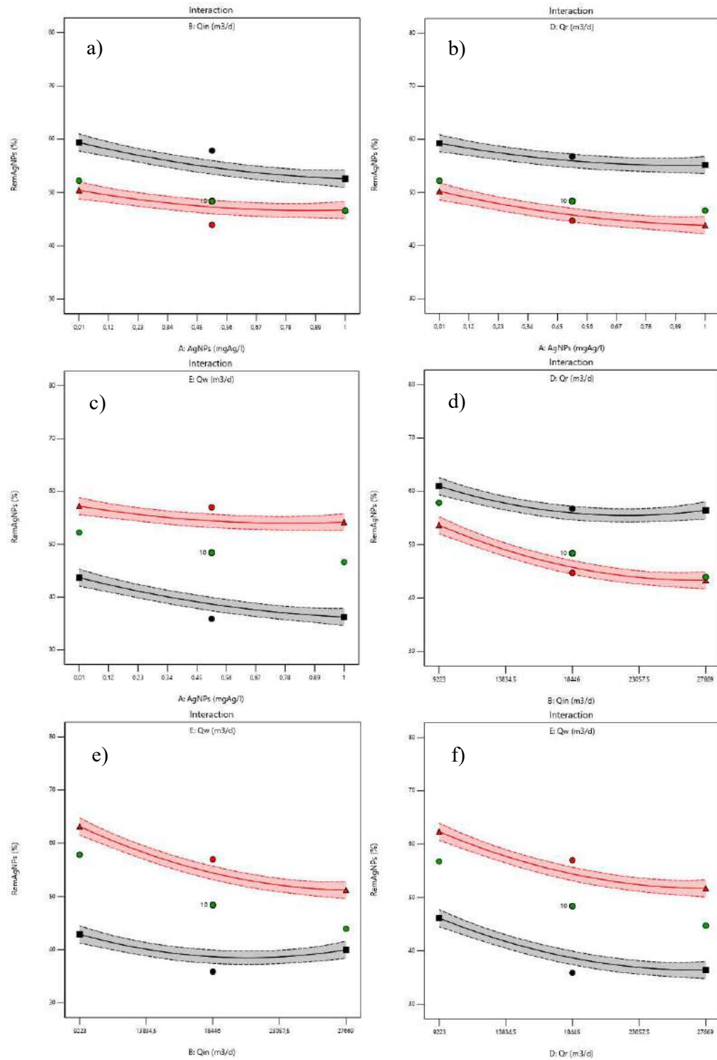
Figura 6.4 - Gráficos de las interacciones más significativas entre los factores: a) AB, b) AD, c) AE, d) BD, e) BE y f) DE, para la respuesta 'R1: Remoción de AgNPs' en el modelo BSM1 modificado.
