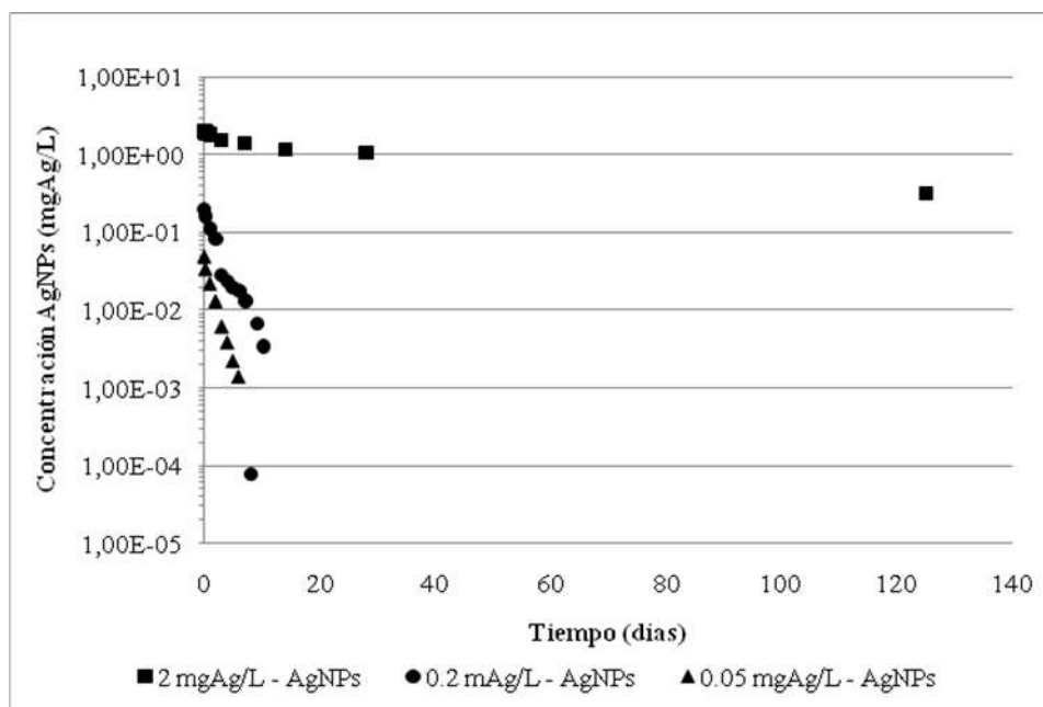
Figura 3.6 - Gráfico de la concentración de AgNPs remanente durante la disolución y liberación de iones plata, para diferentes concentraciones iniciales de AgNPs (2; 0,2; 0,05 mg Ag/L).
