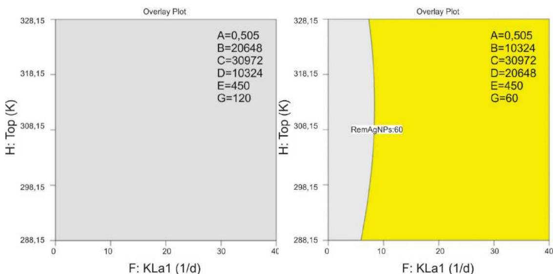
Figura A.30 - Zona óptima de las respuestas analizadas para el modelo BSM2 modificado. Escenario 3. Remoción de AgNPs 60%. Factores F: KLa1 y H: Top. A: 0,505mgAg/L, C: 30972 m 3 /d, E: 450 m 3 /d. En a) B: 20648 m 3 /d, D: 10324m 3 /d, G: 120 1/d, b) B: 10324 m 3 /d, D: 20648 m 3 /d, G: 60 1/d.
