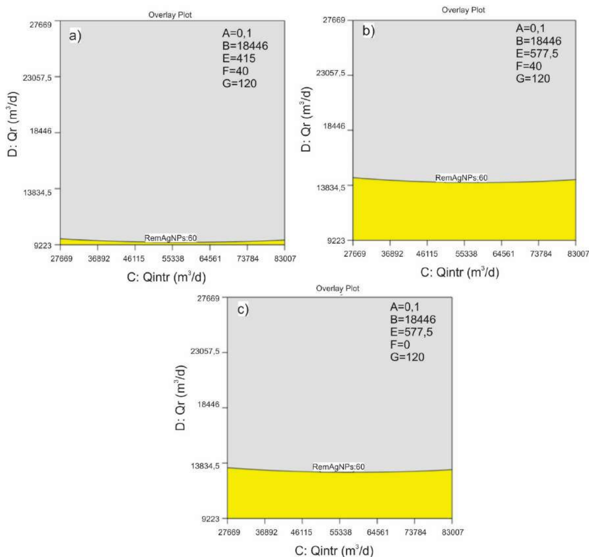
Figura 6.15 - Zona óptima de las respuestas analizadas para modelo BSM1 modificado. Remoción de AgNPs 60%. Factores C: caudal de reciclo interno ( \text{m}^3/\text{d} ), D: Caudal de reciclo ( \text{m}^3/\text{d} ). A: 0,1 \text{ mgAg/L} , B: 18446 \text{ m}^3/\text{d} , G: 120 \text{ 1/d} . En a) E: 415 \text{ m}^3/\text{d} , F: 40 \text{ 1/d} , b) E: 577,5 \text{ m}^3/\text{d} , F: 40 \text{ 1/d} , c) E: 577,5 \text{ m}^3/\text{d} , F: 0 \text{ 1/d} .
