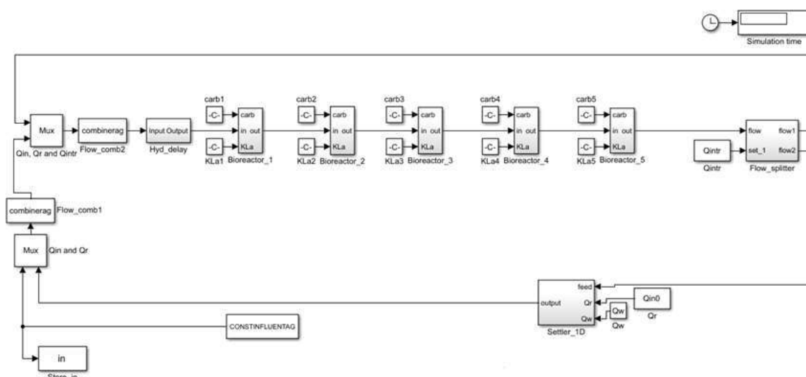
Figura 4.5 - Vista de captura de pantalla del modelo BSM1 modificado en MATLAB/Simulink®, archivo openloopag.mdl .
