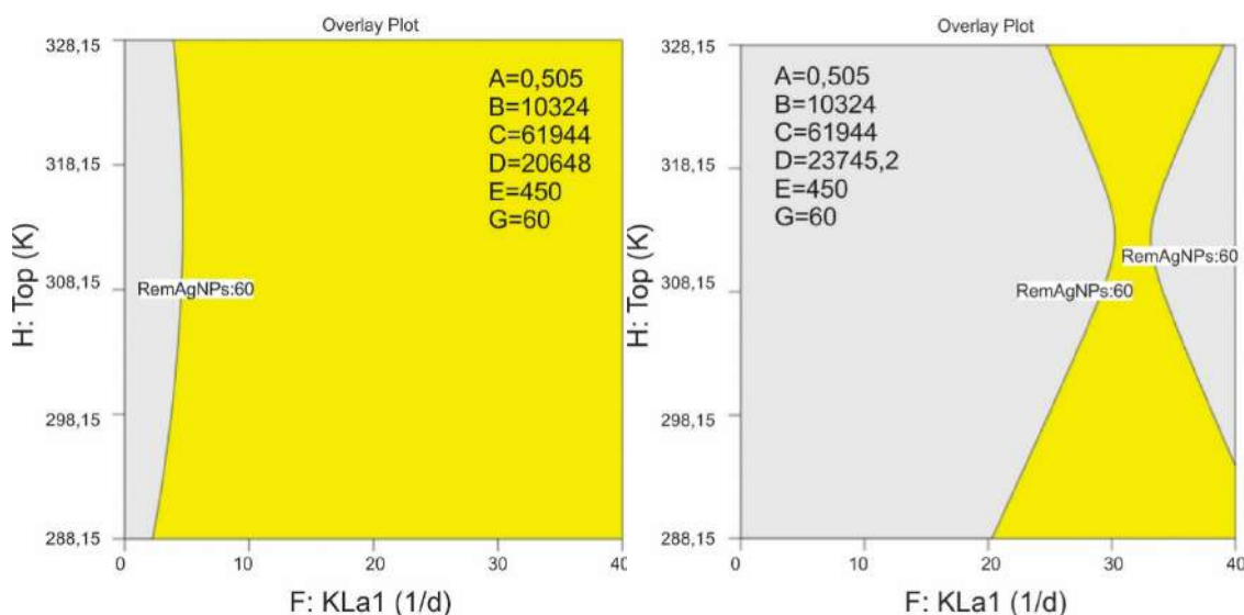
Figura A.31 - Zona óptima de las respuestas analizadas para el modelo BSM2 modificado. Escenario 3. Remoción de AgNPs 60%. Factores F: KLa1 y H: Top. A: 0,505mgAg/L, B: 10324 m 3 /d, C: 61944 m 3 /d, E: 450 m 3 /d, G: 60 1/d. En a) D: 20648 m 3 /d, b) D: 23745,2 m 3 /d.
