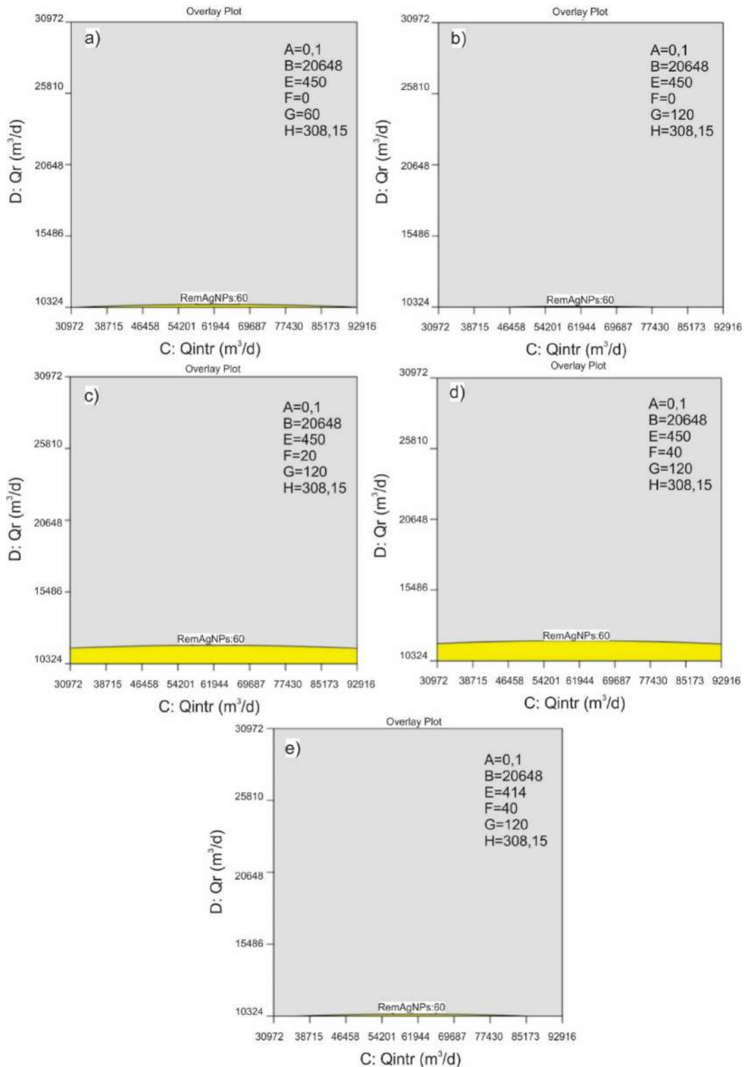
Figura 6.31 - Zona óptima de las respuestas analizadas para el modelo BSM2 modificado. Remoción de AgNPs 60%. Factores C: Qintr y D: Qr. A: 0,1 mgAg/L, B: 20648 m³/d, H: 308,15 K. En a) E: 450 m³/d, F: 0 l/d, G: 60 l/d, b) E: 450 m³/d, F: 0 l/d, G: 120 l/d, c) E: 450 m³/d, F: 20 l/d, G: 120 l/d, d) E: 450 m³/d, F: 40 l/d, G: 120 l/d, e) E: 414 m³/d, F: 40 l/d, G: 120 l/d.
