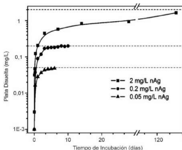
Figura 3.5 - Gráfico de disolución de plata como ión plata en el largo plazo, para distintas concentraciones iniciales de AgNPs (2; 0,2 y 0,05 mg/L) de 2 nm de diámetro a temperatura ambiente, en ausencia de luz (Liu & Hurt, 2010).
