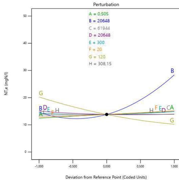
Figura 6.27 - Gráfico de perturbaciones para R4: NT, en el modelo BSM2 modificado.
