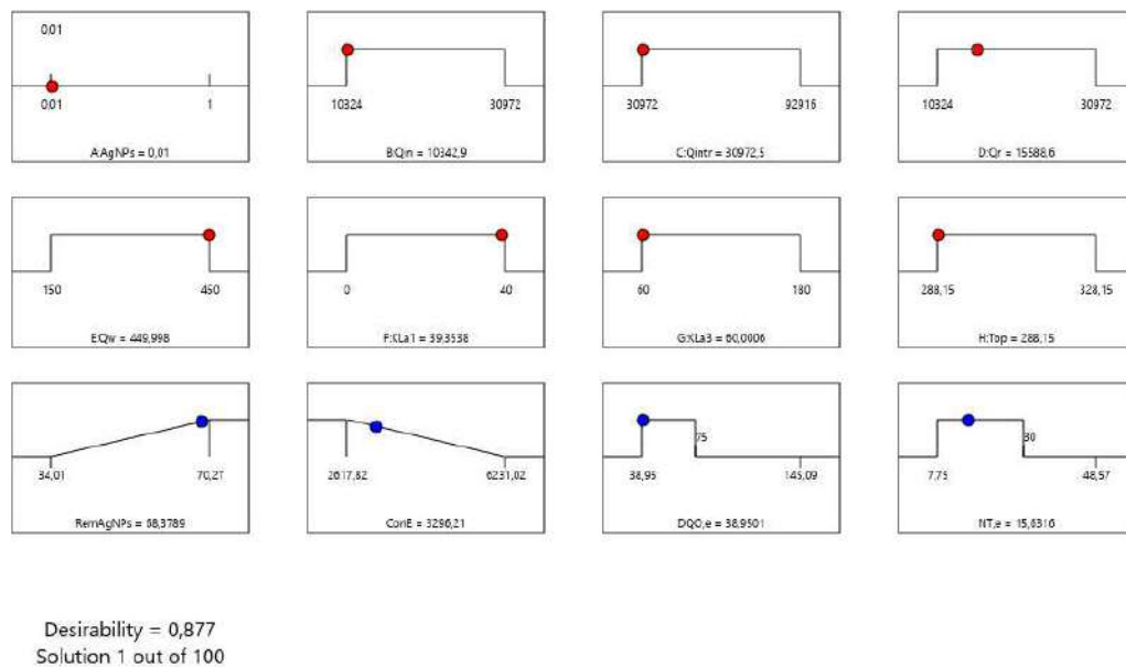
Figura A.19 - Optimización numérica para el Escenario 1-A, para el modelo BSM2 modificado. AgNPS: 0,01 mgAg/L, Qin libre. Deseabilidad: 0,877.
