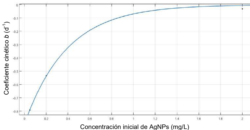
Figura 3.7 - Gráfico del ajuste del coeficiente de disolución de AgNPs en función de la concentración inicial de AgNPs.
