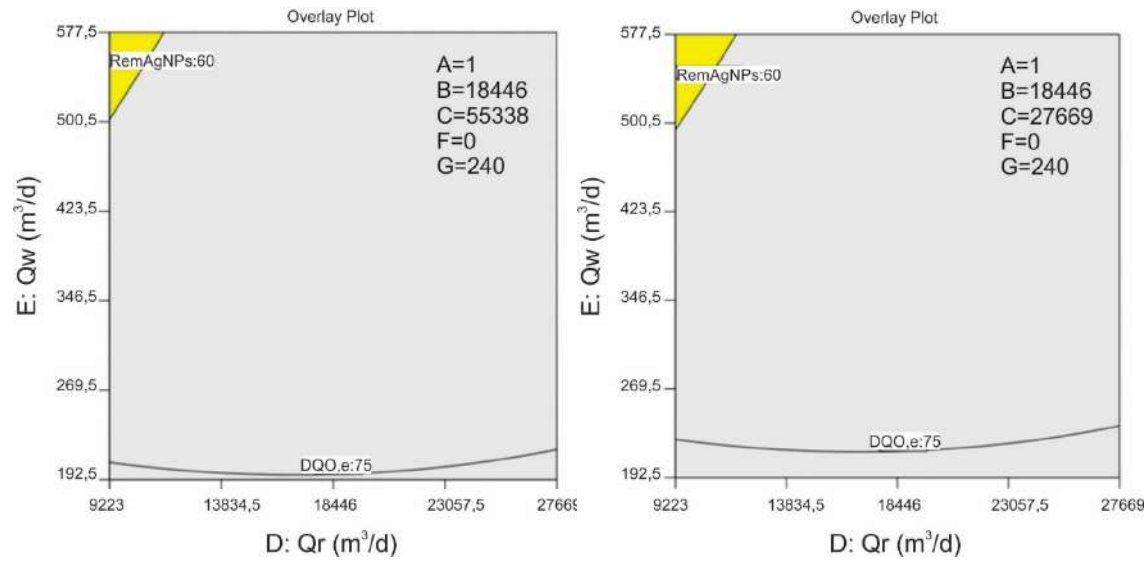
Figura A.17 - Zona óptima de las respuestas analizadas para el modelo BSM1 modificado. Escenario 4. Remoción de AgNPs 60%. Factores D: Qr y E: Qw. A:1 mgAg/L, B: 18446 m³/d, F: 0 l/d, G: 240 l/d. En a) C: 55338 m³/d, b) C: 27669 m³/d.
