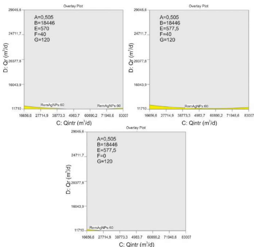
Figura A.9 - Zona óptima de las respuestas analizadas para el modelo BSM1 modificado. Escenario 3. Remoción de AgNPs 60%. Factores C: Qintr y D: Qr. A: 0,505mgAg/L, B: 18446 m³/d, G: 120 l/d. En a) E: 570 m³/d, F: 40 l/d, b) E: 577,5 m³/d, F: 40 l/d c) E: 577,5 m³/d, F: 0 l/d.
