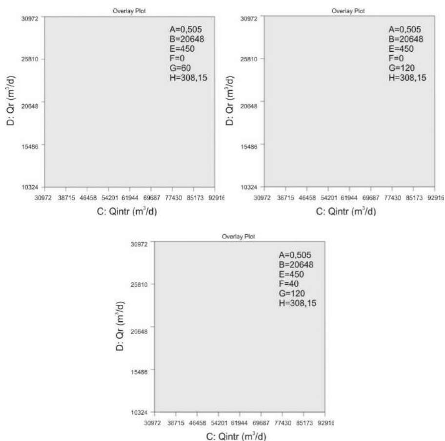
Figura A.27 - Zona óptima de las respuestas analizadas para el modelo BSM2 modificado. Escenario 3. Remoción de AgNPs 60%. Factores C: Qintr y D: Qr. A: 0,505mgAg/L, B: 20648 m³/d, E: 450 m³/d, H: 308,15 K. En a) F: 0 1/d, G: 60 1/d, b) F: 0 1/d, G: 120 1/d, c) F: 40 1/d, G: 120 1/d.
