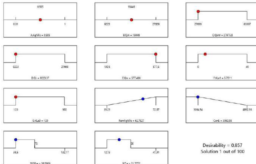
Figura A.8 - Optimización numérica para el Escenario 3-B., para el modelo BSM1 modificado. AgNPS: 0,505mgAg/L, Qin: 18446 m 3 /d. Deseabilidad: 0,857.
