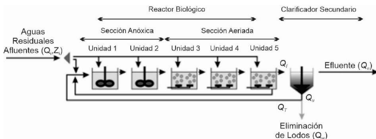
Figura 4.1 - Representación esquemática de la planta para el modelo BSM1. Adaptado de Gernaey et al. (2014) y Alex et al. (2009a). Consiste en un tratamiento biológico que incluye dos reactores anóxicos (Unidades 1 y 2) y tres aeróbicos (Unidades 3, 4 y 5), seguidos por un sedimentador secundario.
