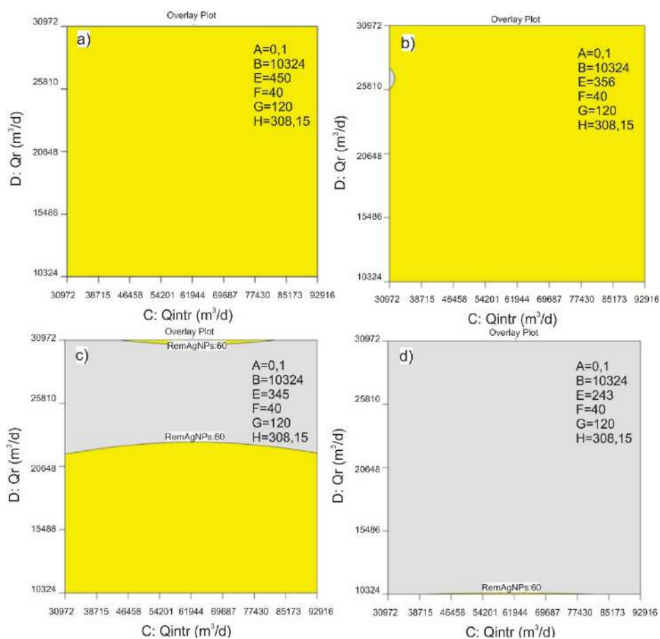
Figura 6.32 - Zona óptima de las respuestas analizadas para modelo BSM2 modificado. Remoción de AgNPs 60%. Factores C: Qintr y D: Qr. A: 0,1 mgAg/L, B: 10324 m 3 /d, F: 40 1/d, G: 120 1/d H: 308,15 K. En a) E: 450 m 3 /d, b) E: 356 m 3 /d, c) E: 345 m 3 /d, d) E: 234m 3 /d.
