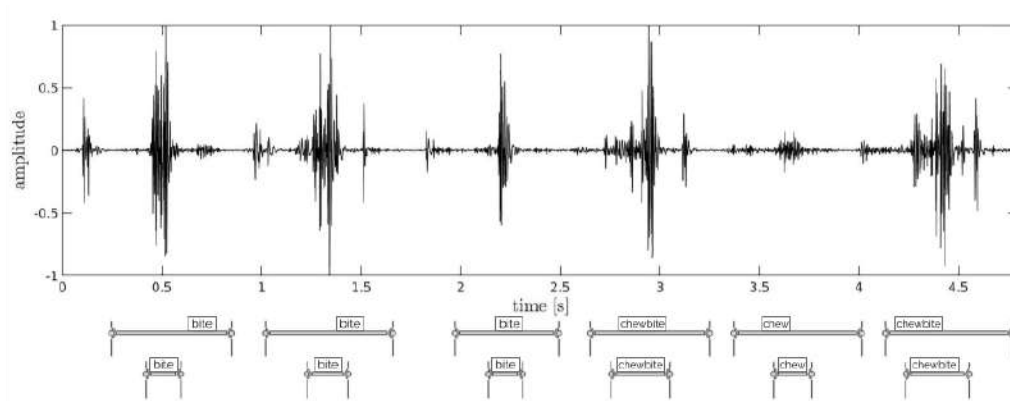
Figura 2.4: Comparación visual de un ejemplo de una señal con etiquetas originales (arriba) y etiquetas erosionadas (abajo) con delimitadores temporales (la escala de tiempo en la parte superior está expresada en segundos).
