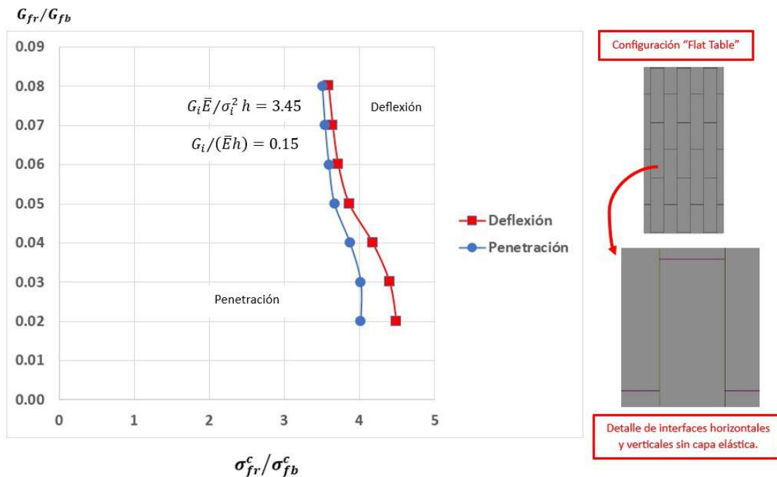
Figura C.9: Curvas de mecanismos de deflexión y penetración para configuración Flat Table.
