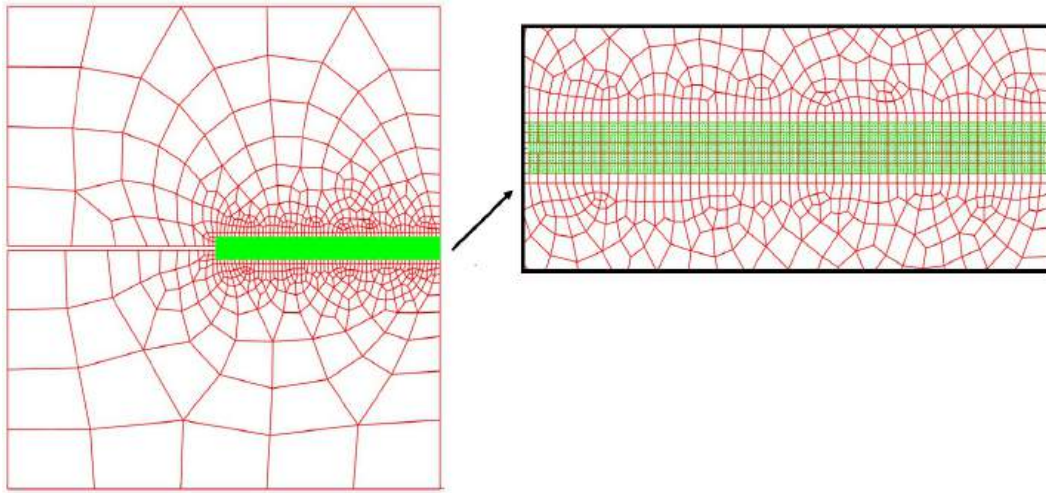
Figura 6.2: Discretización para aplicación del método Ov-IEFG-FEM empleando el modelo de campo de fase. Los cálculos mediante FEM se llevan a cabo en la malla gruesa de color rojo, mientras que los cálculos del IEFG se hacen a través de la distribución fina de nodos representados por los puntos de color verde.
