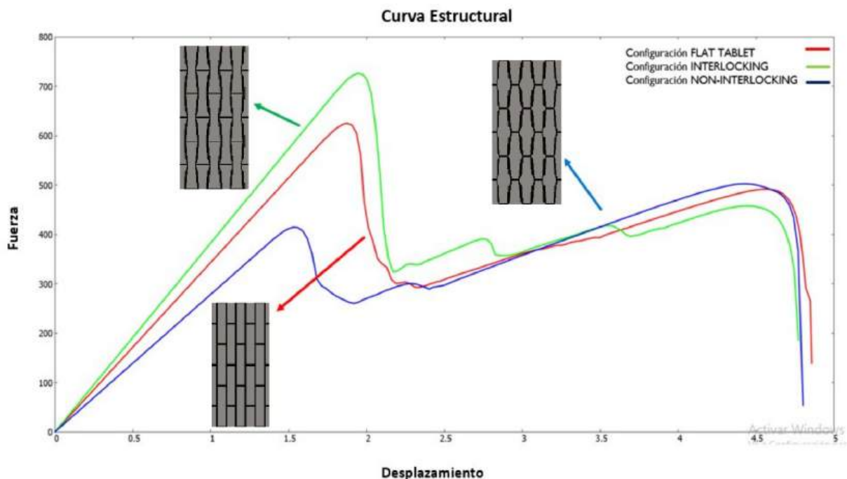
Figura 4.3: Respuesta numérica de las configuraciones Tableta Plana (Flat Table), Entrelazada (Interlocking) y No Entrelazada (Non-Interlocking)
