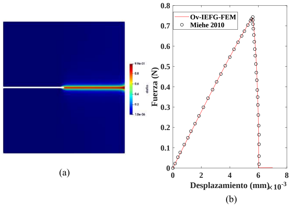
Figura 6.3: (a) Evolución del campo de fase en muestra tipo SENT. (b) Curva Fuerza vs Desplazamiento para muestra tipo SENT.
