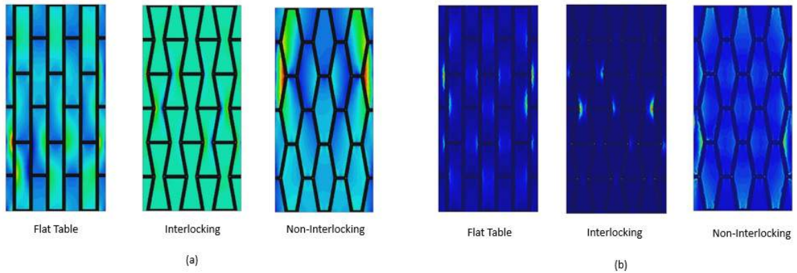
Figura C.8: (a) Distribución de tensiones \sigma_{yy} en las configuraciones Flat Table, Interlocking, Non-Interlocking, (b) Evolución del daño (Phase-Field) en las configuraciones Flat Table, Interlocking, Non-Interlocking
