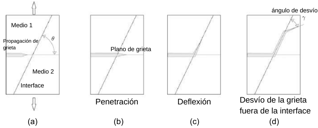
Figura 3.2: Modos de interacción entre una grieta en propagación que impacta sobre una interface con un ángulo \theta . (a) Esquema del problema. (b) Penetración. (c) Deflexión. (d) Desvío de la grieta fuera de la interface.
