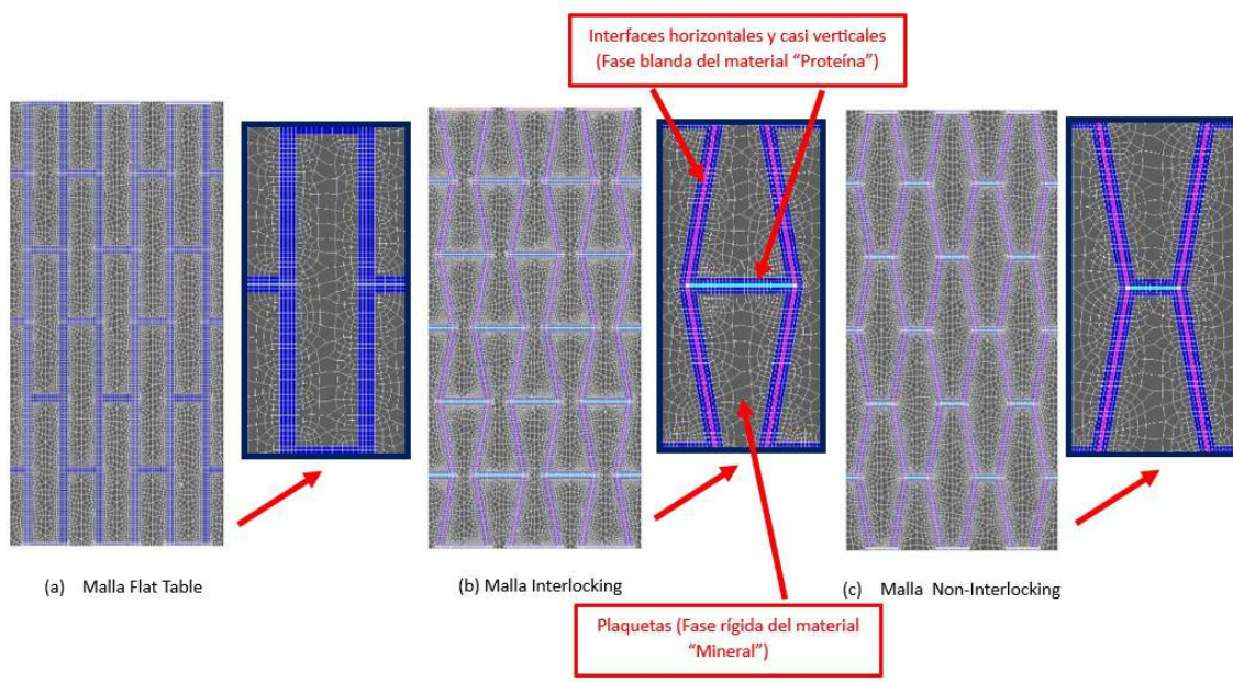
Figura C.5: (a) Malla y celda unitaria para la configuración Flat Table, (b) Malla y celda unitaria para la configuración Interlocking y (c) Malla y celda unitaria para la configuración Non-Interlocking.
