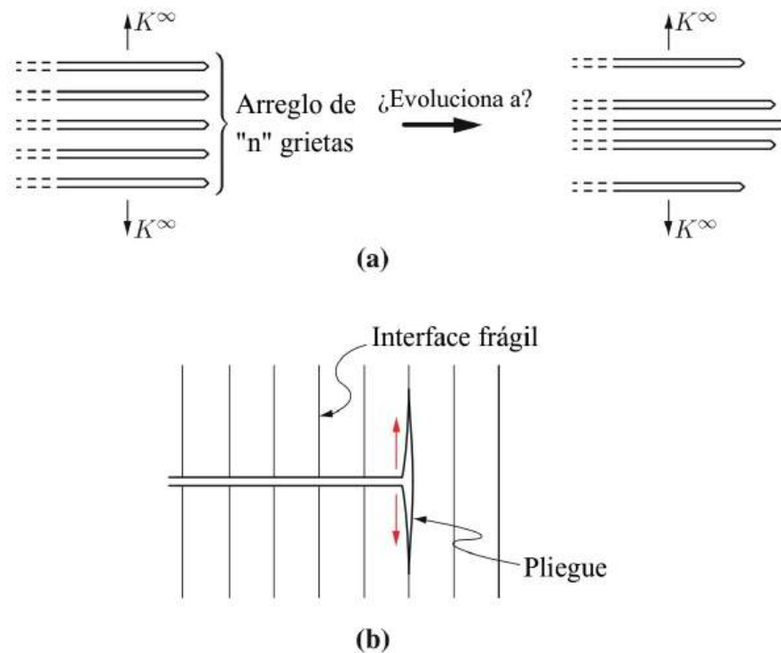
Figura 4.1: Representación esquemática de los posibles mecanismos de aumento de tenacidad: a) Multiplicación de grietas; b) Desviación de grietas en sólidos laminados a lo largo de una interface frágil.
