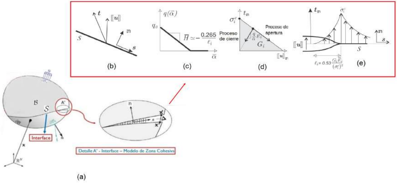
Figura 3.1: (a) Esquema de un cuerpo con una interface cohesiva. (b) Vectores de tracción t y separación \llbracket u \rrbracket en la interface. (c) Ley de ablandamiento, q(\bar{\alpha}) que gobierna la degradación tracción-separación. (d) Ley tracción-separación para la apertura de una interface en el modo I. El área bajo la curva es igual a la energía de fractura G_i y la componente de máxima tensión es \sigma_i^c . (e) Estimación de la longitud característica cohesiva \ell_i
