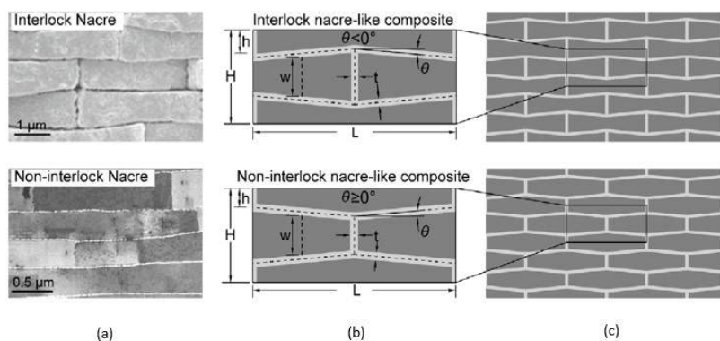
Figura C.4: (a) Imagen de Hyriopsis Cumingii con configuración entrelazada (Interlocking), (b) Parámetros geométricos ( H, h, L, w, t en mm y \theta en grados) de celdas unitarias, (c) Configuraciones Interlocking y Non-Interlocking para estructura tipo nácar.
