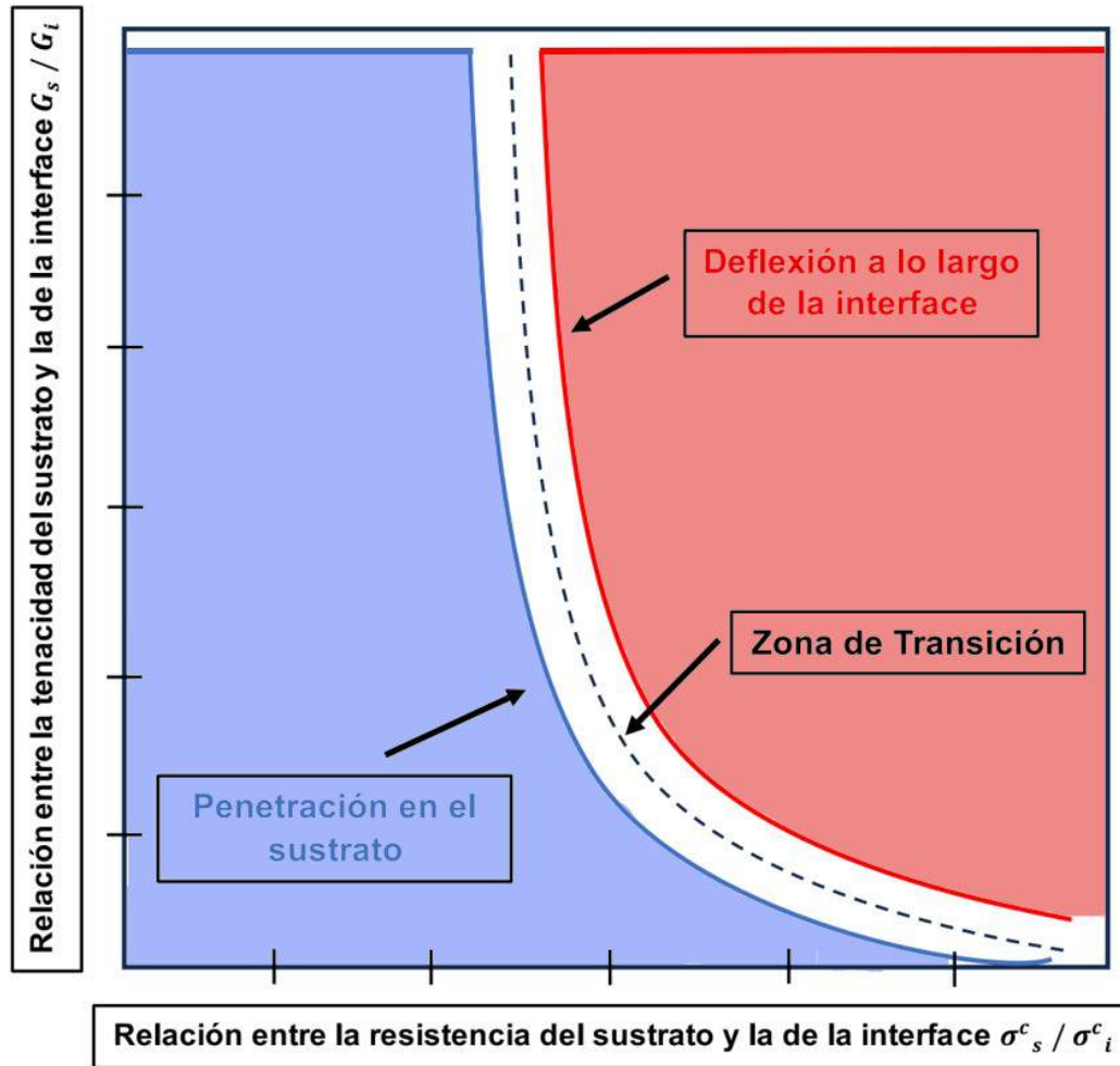
Figura 3.3: Comportamiento esquemático de mecanismos de penetración y deflexión de una grieta propagante que incide en una interface que forma \theta = 90^\circ con respecto a la dirección de propagación de la grieta.
