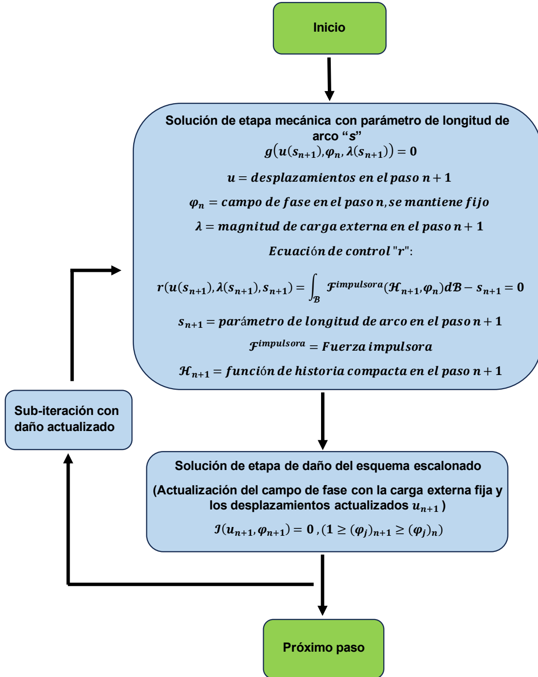
Figura 5.1: Representación esquemática de la estrategia de longitud de arco propuesta con un esquema escalonado explícito.
