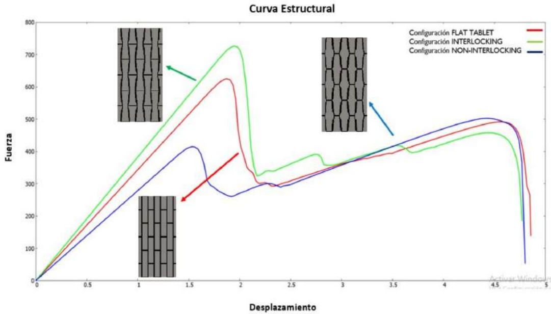
Figura C.7: Curvas estructurales para las configuraciones: Flat Table, Interlocking y Non-Interlocking.
