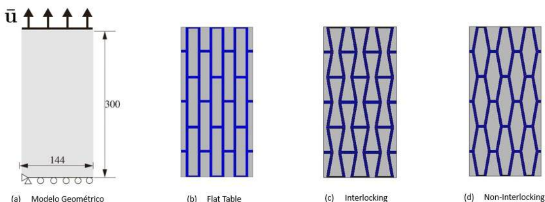
Figura C.3: Estructuras compuestas tipo nácar: (a) Dimensiones de la geometría y condiciones de borde aplicadas, (b) Configuración Flat Table, (c) Configuración Interlocking, (d) Configuración Non-Interlocking.
