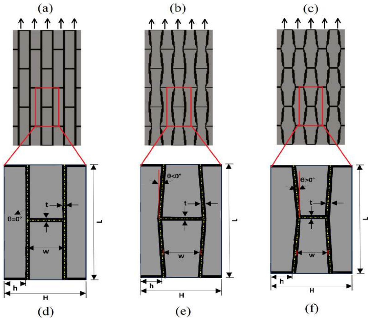
Figura 4.5: (a) Configuración geométrica Tableta Plana (Flat Table), (b) Configuración geométrica Entrelazada (Interlocking), (c) Configuración geométrica No Entrelazada (Non-Interlocking), (d-f) Parámetros geométricos ( H, h, L, w, t en mm y \theta en grados) de celdas unitarias para las configuraciones Tableta plana, Entrelazada y No Entrelazada para la estructura tipo nácar.
