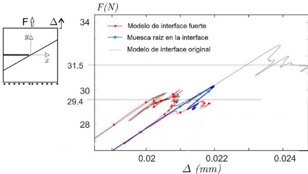
Figura 3.4: Comparación de pruebas para el análisis del incremento de tenacidad de una muestra.
