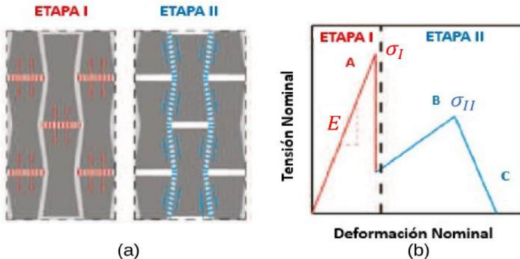
Figura 4.2: (a) Deformación teórica por etapas de las interfaces, (b) Curva teórica tensión-deformación dividida por etapas de deformación
