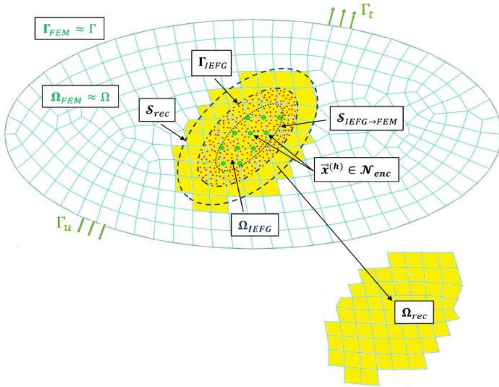
Figura 6.1: Representación del dominio del problema para una solución numérica empleando el método Ov-IEFG-FEM.
