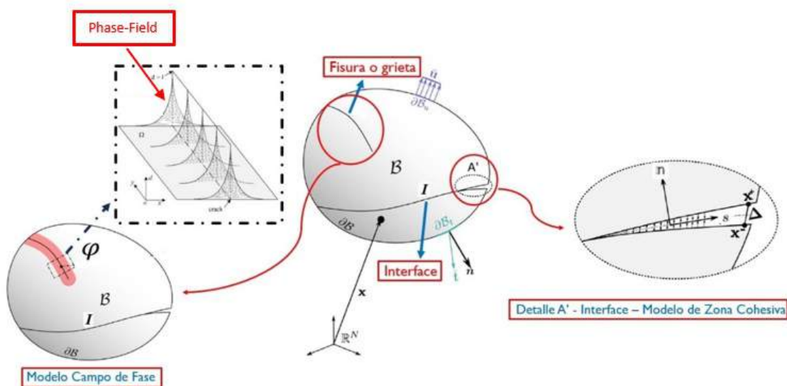
Figura C.1: Esquema de modelado mecánico aplicado en la implementación numérica.
