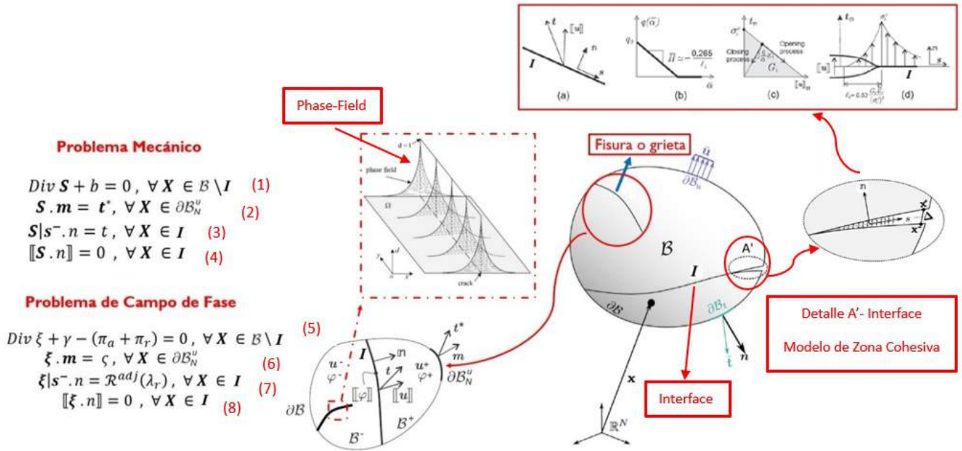
Figura C.2: Ecuaciones gobernantes para los problemas mecánico y de campo de fase aplicadas en la fase rígida del material de los diseños bioinspirados y descripción esquemática del modelo de interface de superficie cohesiva aplicado a la fase blanda del material.
