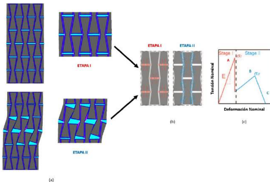
Figura C.6: Proceso de deformación para la configuración Interlocking: (a) Mecanismo de falla de las interfaces obtenida de la simulación numérica, (b) Deformación teórica por etapas de las interfaces, (c) Curva teórica de tensión-deformación clasificada por etapas de deformación.
